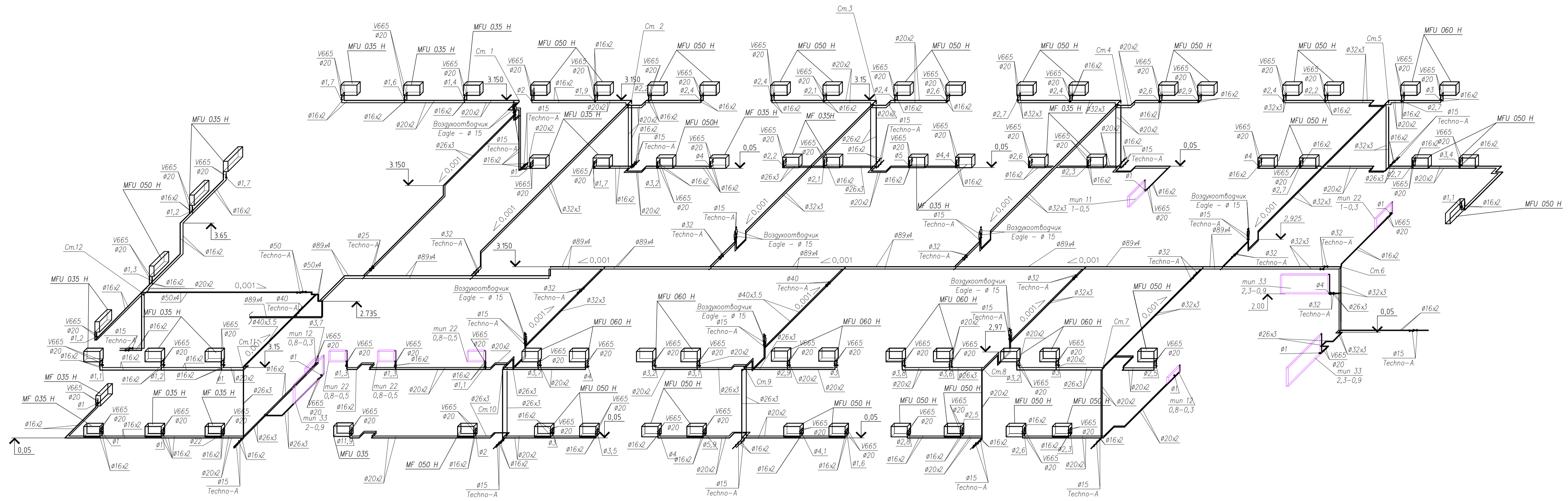
Схема системы отопления
