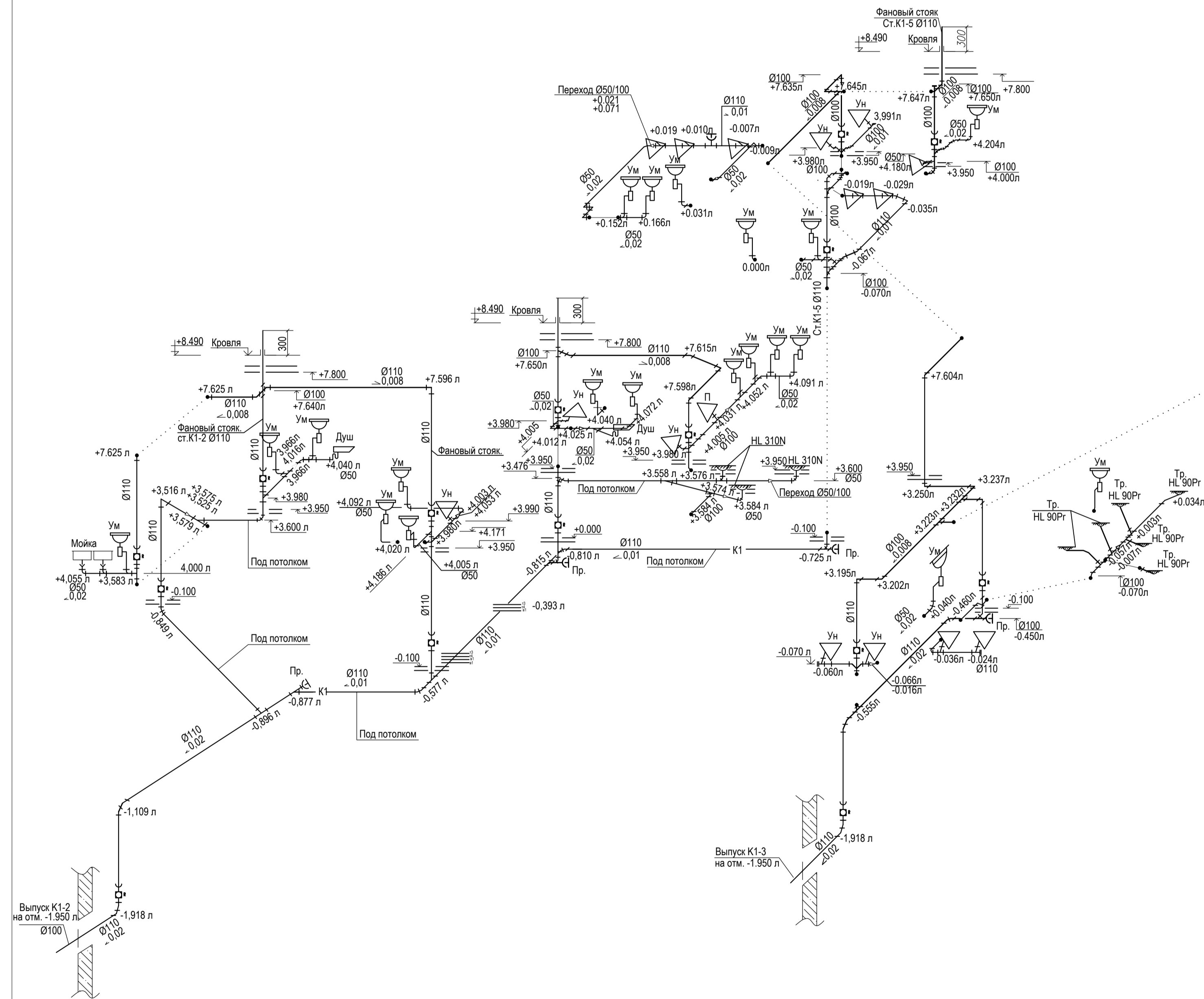
Фрагмент сети в осях 2-6 / В-Ж
