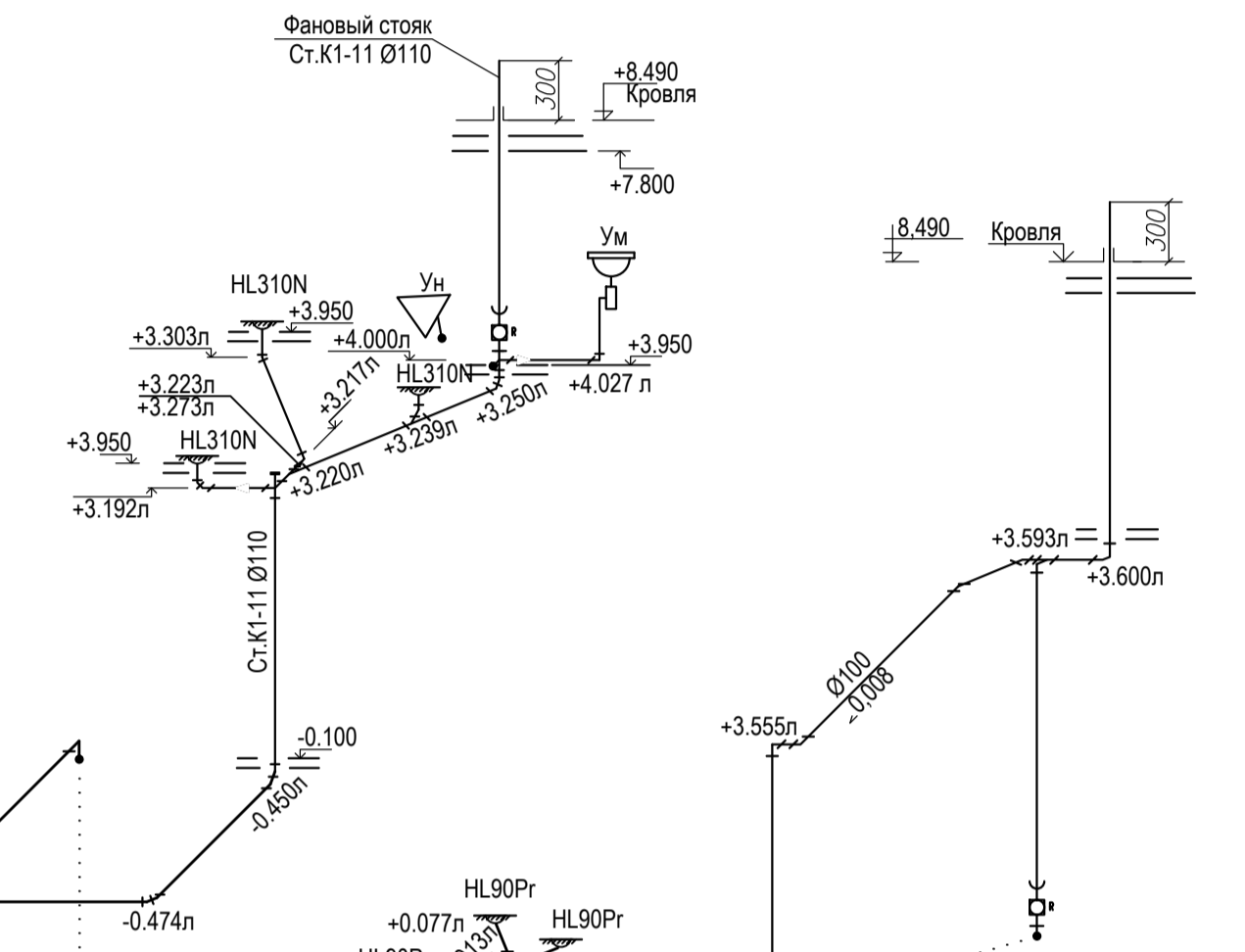
Фрагмент сети в осях 6-12/Б-Е
