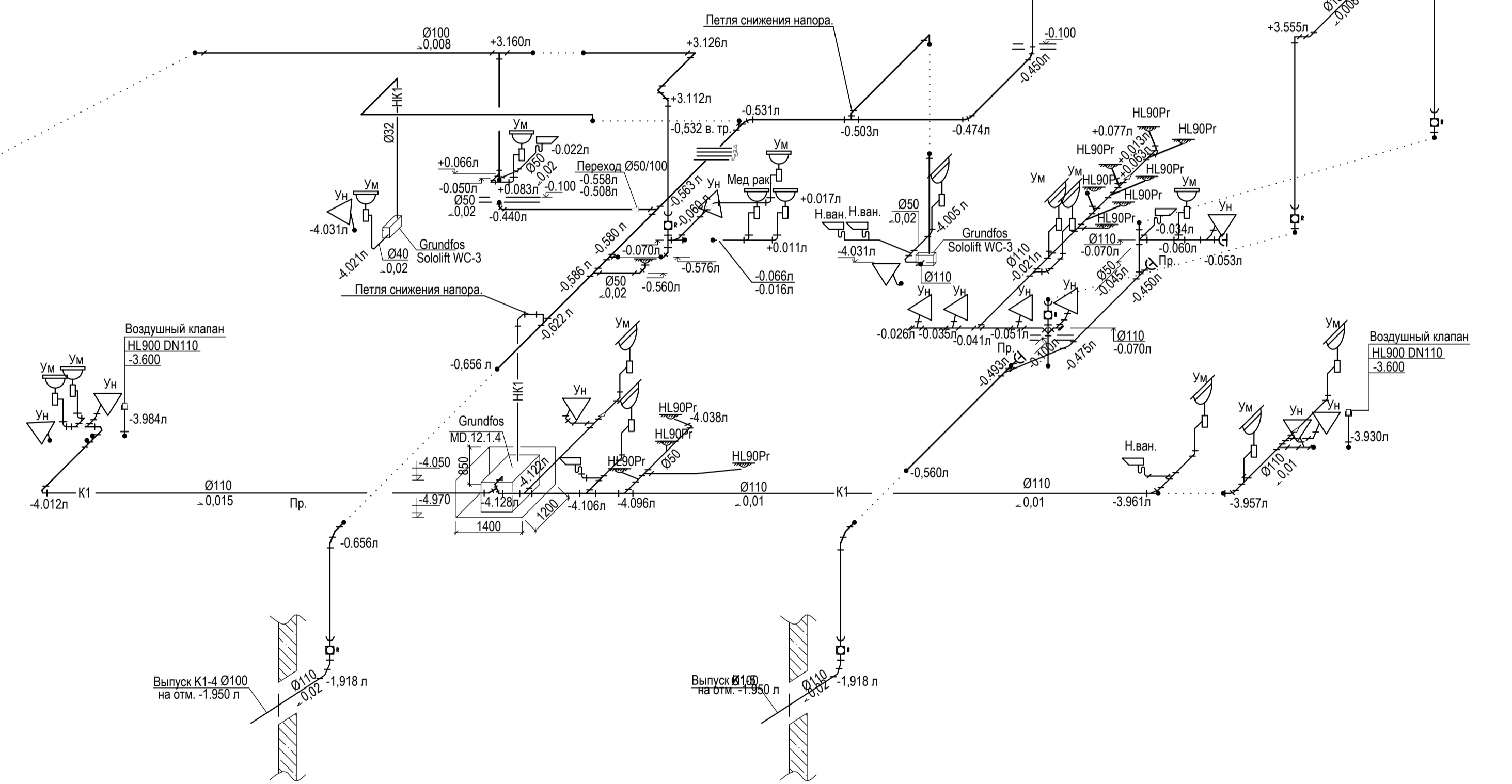
Фрагмент сети в осях 14-22/В-Е
