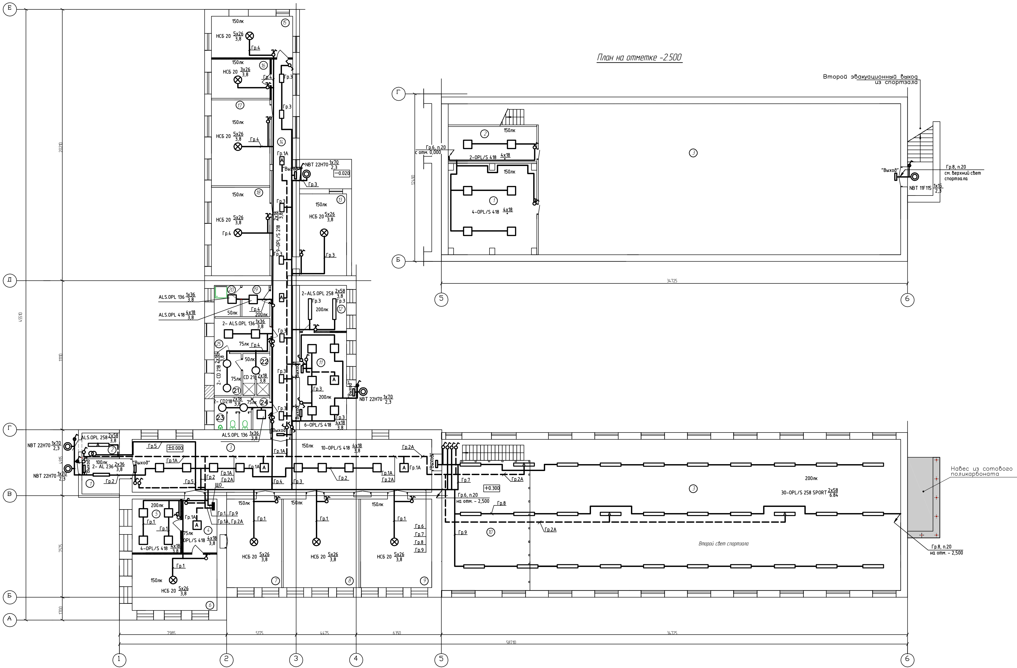
План на отметке ±0.000
