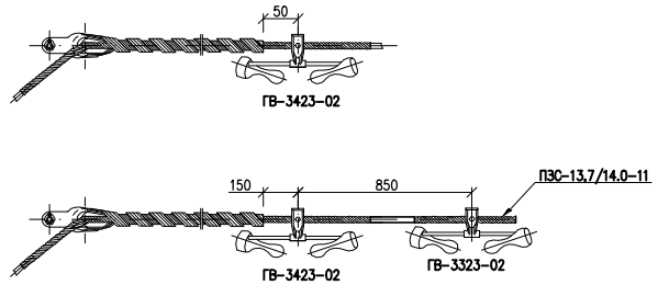
Установка гасителей вибрации на натяжных зажимах
