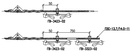
Установка гасителей вибрации на поддерживающих зажимах
