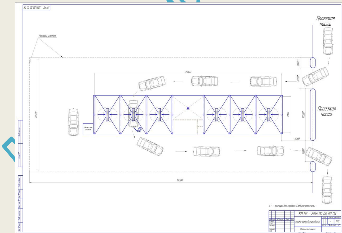
Рисунок 2. План комплекса автомойки (Компас 3D)
