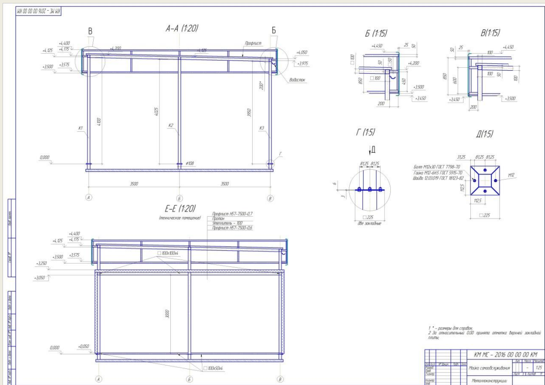
Рисунок 3. Чертеж металлоконструкций каркаса автомойки (Компас 3D)
