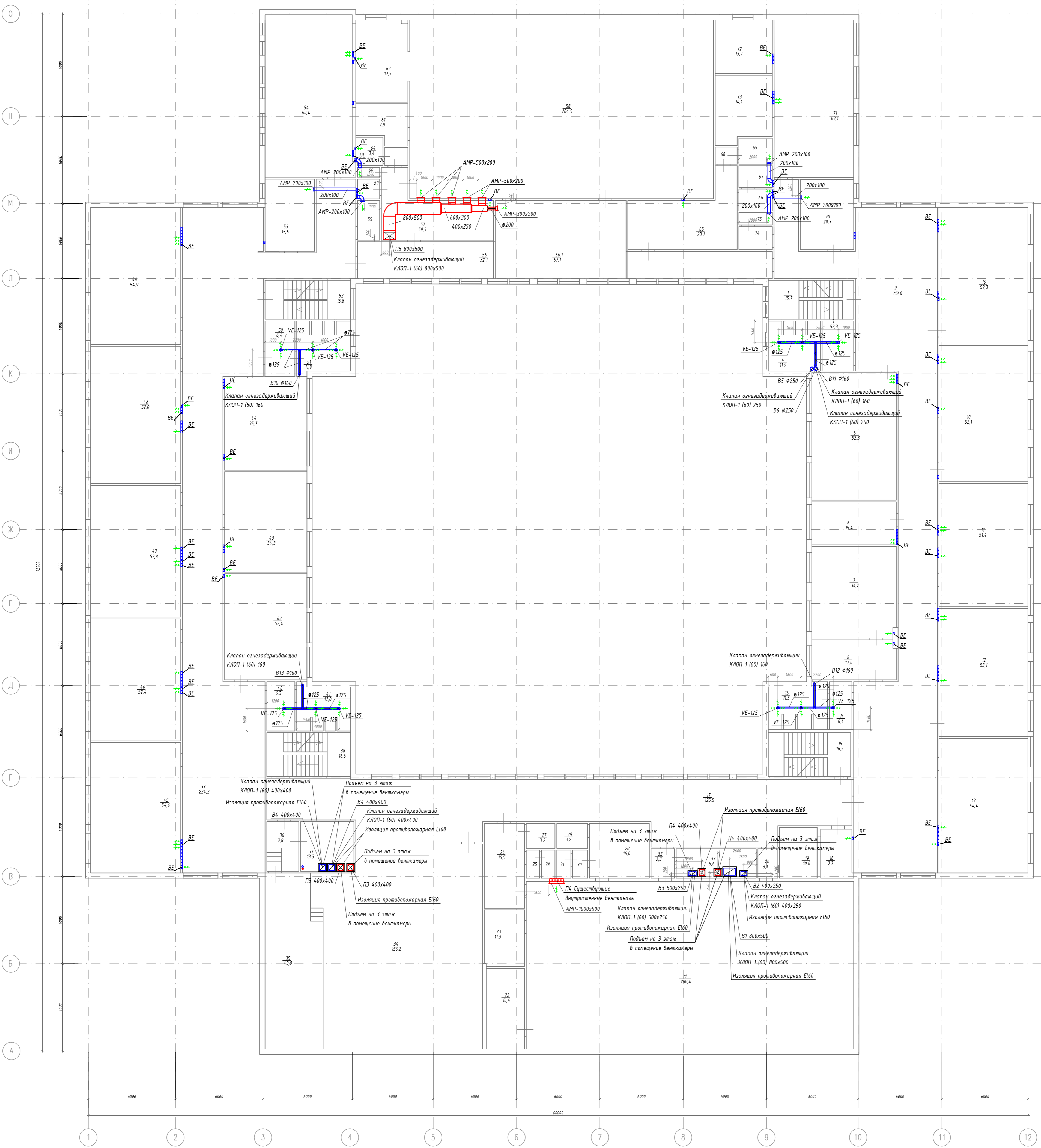
Экспликация помещений
