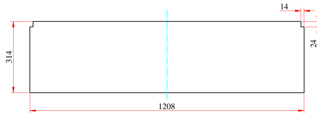
Деталь 7 (1:10)
