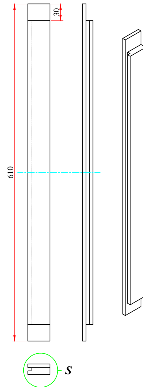
Деталь 2 (1:4)
