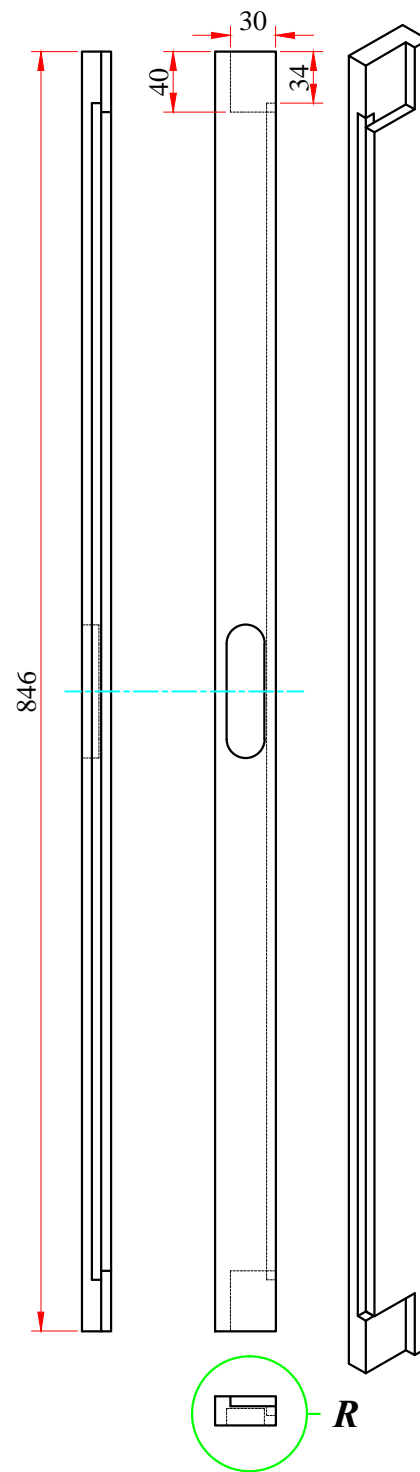
Деталь 1 (1:5)
