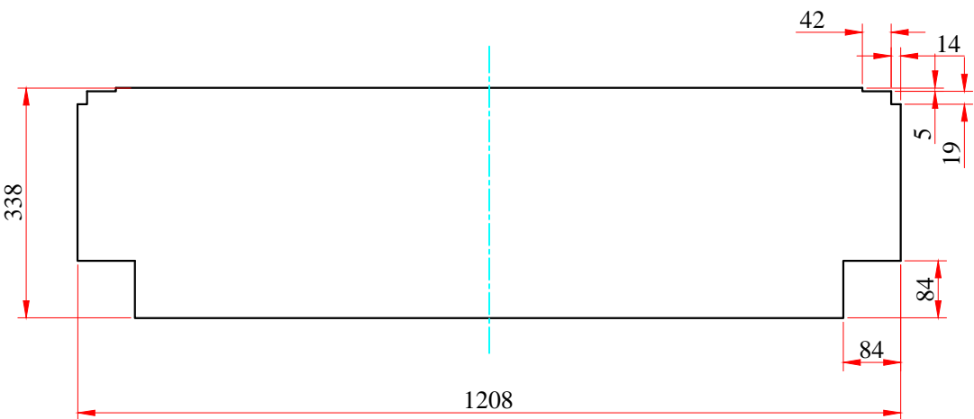
Деталь 8 (1:10)
