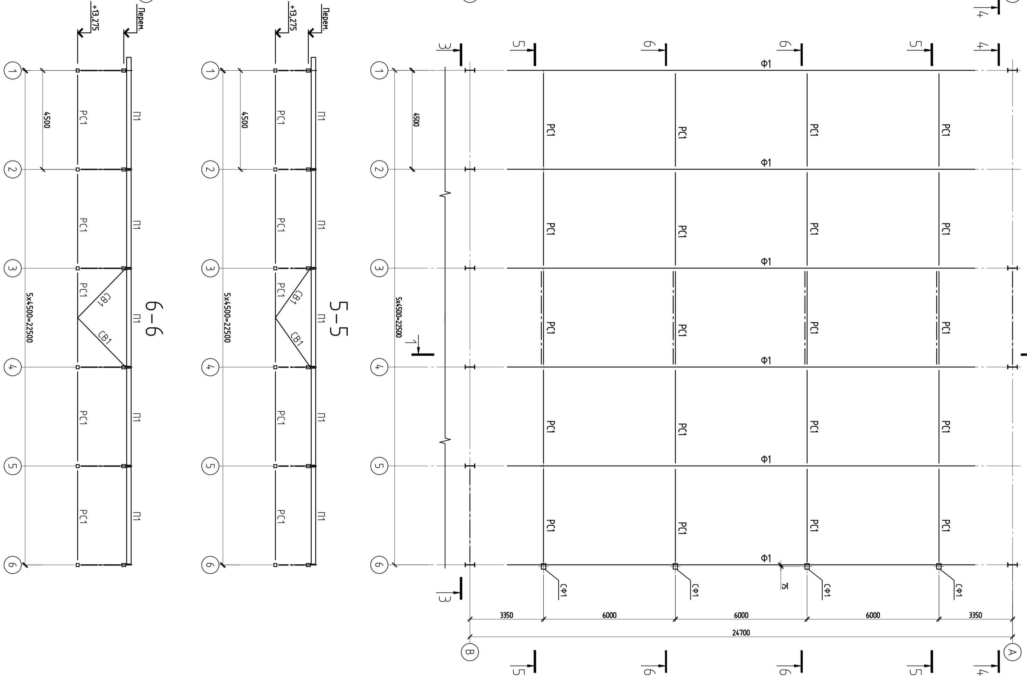
План горизонтальных связей по нижнему поясу ферм
