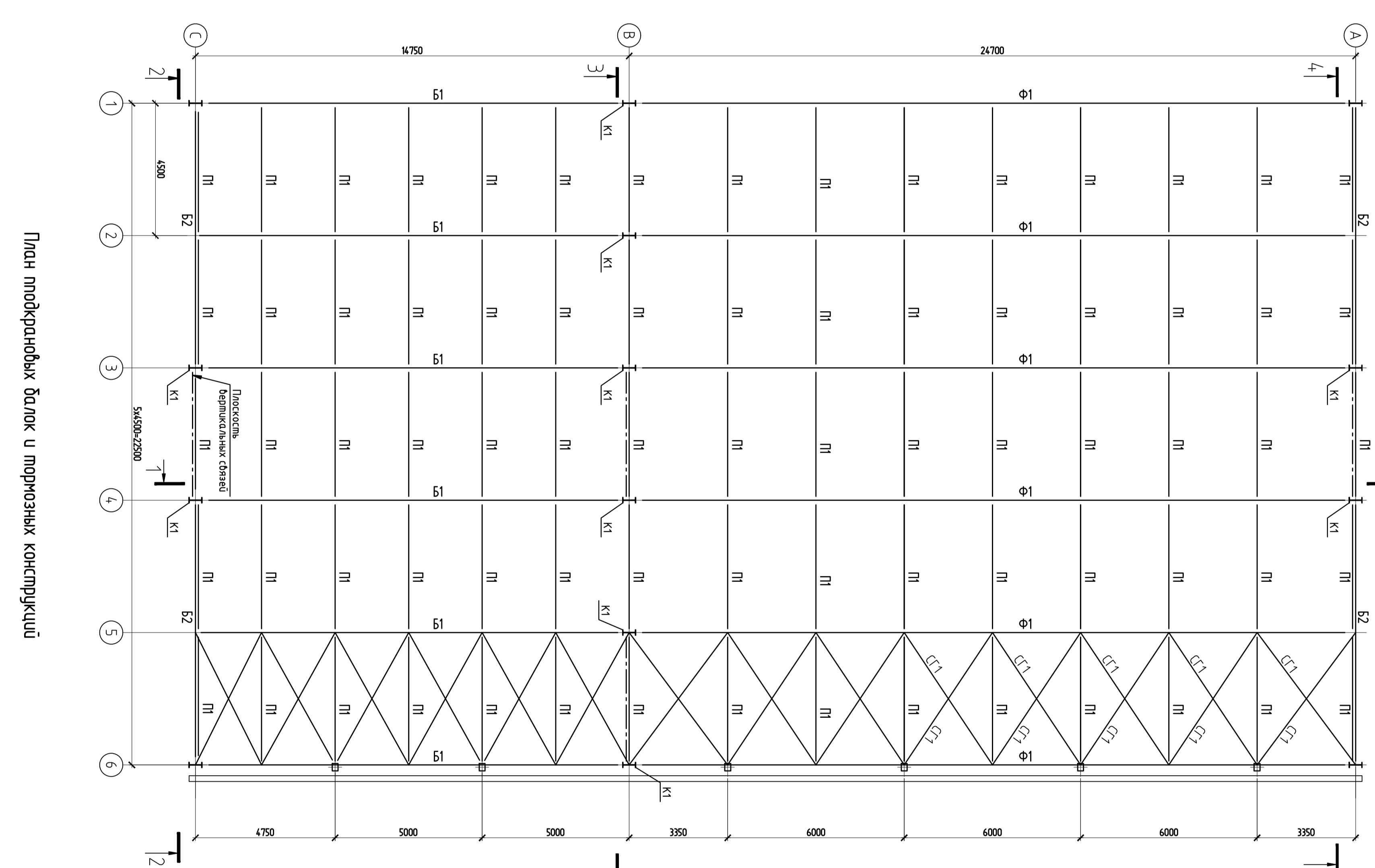
План прогонов и горизонтальных связей по верхнему поясу балок и ферм покрытия
