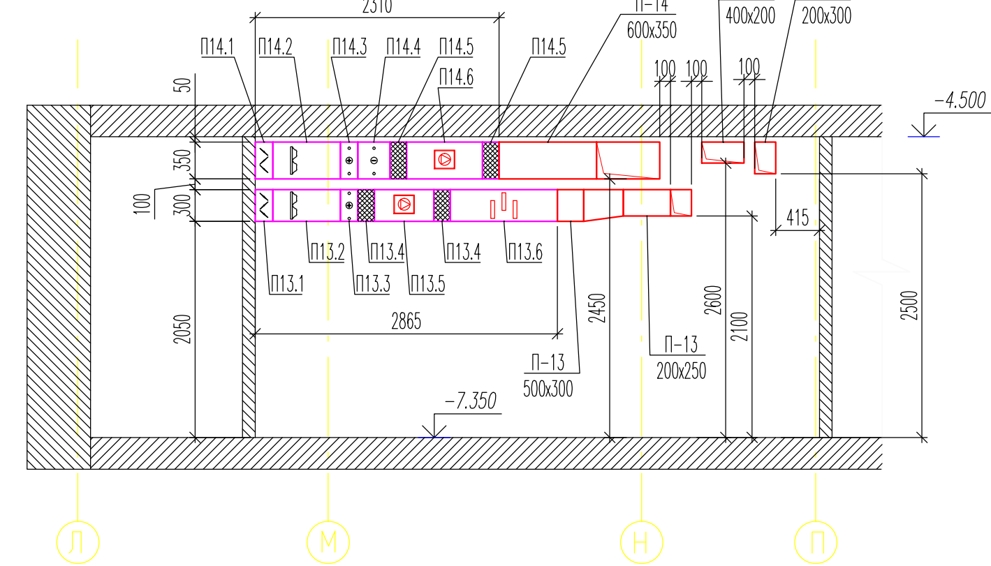
В-В (М 1:50)
