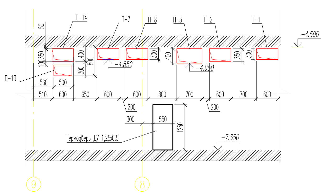
Б-Б (М 1:50)
