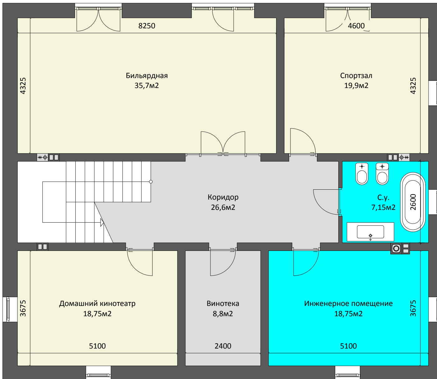
ПЛАН ЦОКОЛЬНОГО ЭТАЖА S пом. этажа = 135,65м 2
