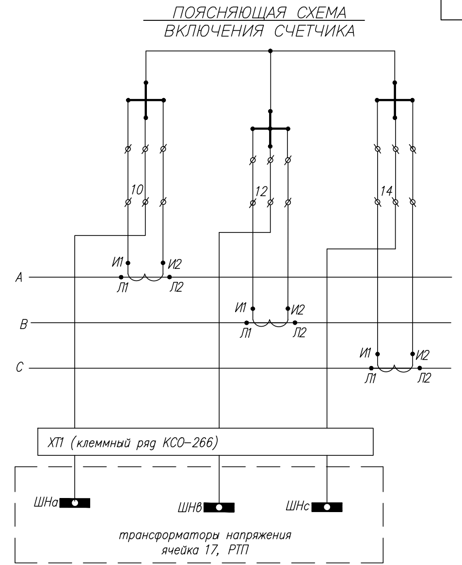
СХЕМА ВКЛЮЧЕНИЯ МЕРКУРИЙ 230 AP
