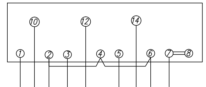
СХЕМА ВКЛЮЧЕНИЯ МЕРКУРИЙ 230 AP
