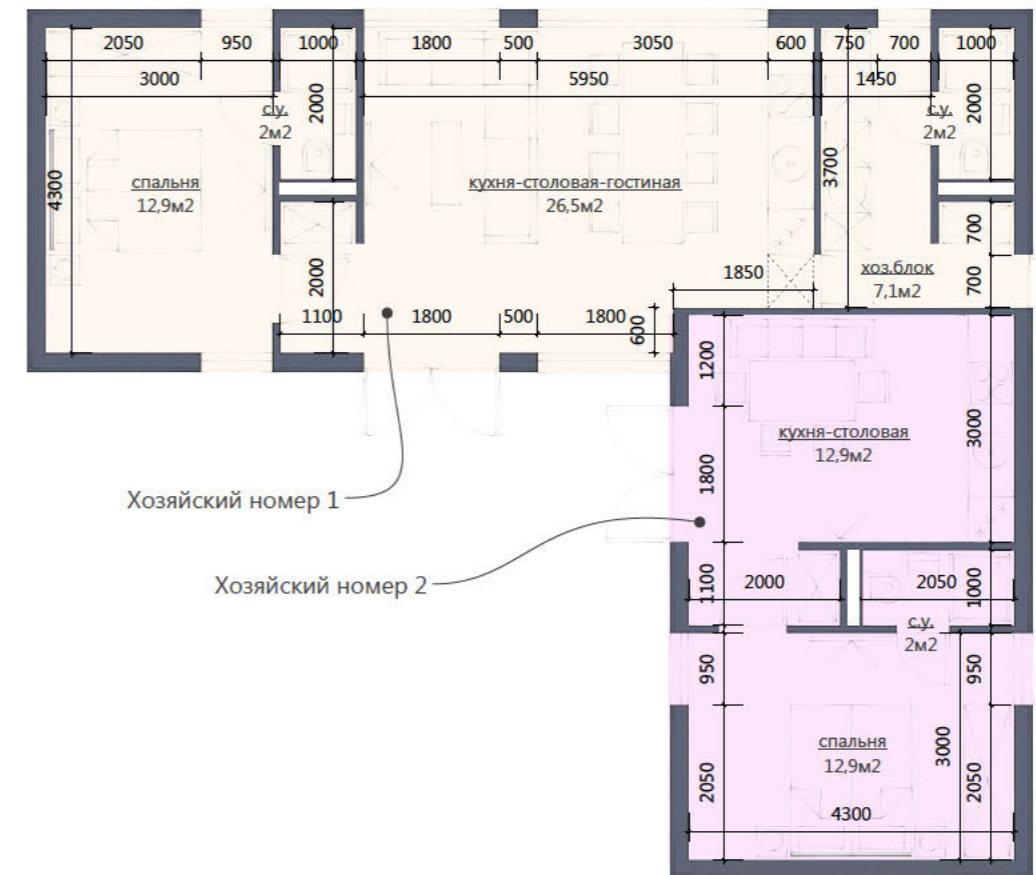
ПЛАН 1-го ЭТАЖА М1:100
