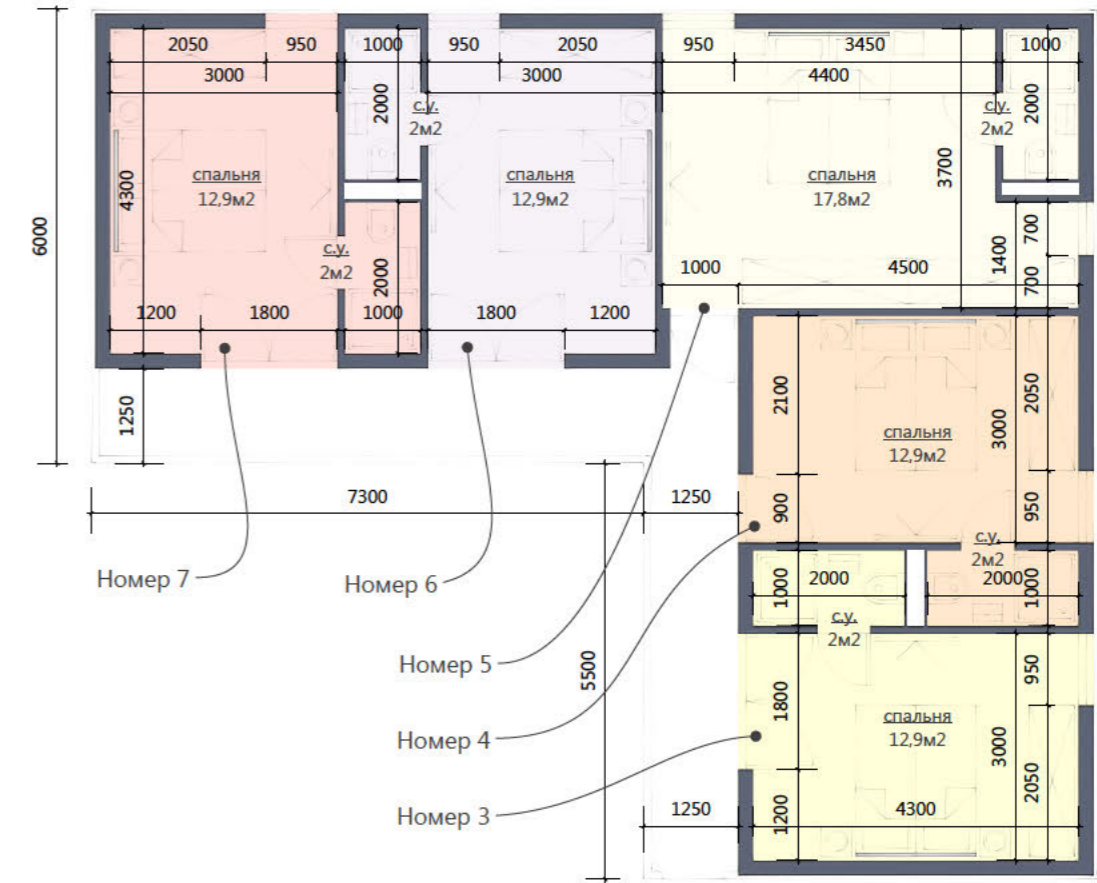
ПЛАН 2-го ЭТАЖА М1:100
