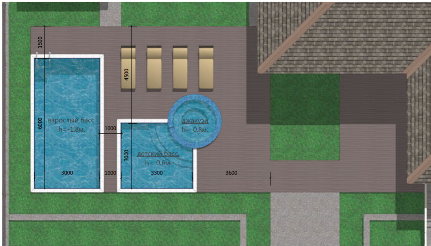
ПЛАН БАСЕЙНА М1:100
