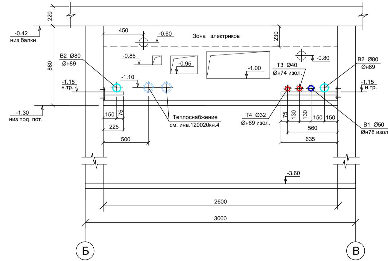
Разрез 1-1 М 1:25
