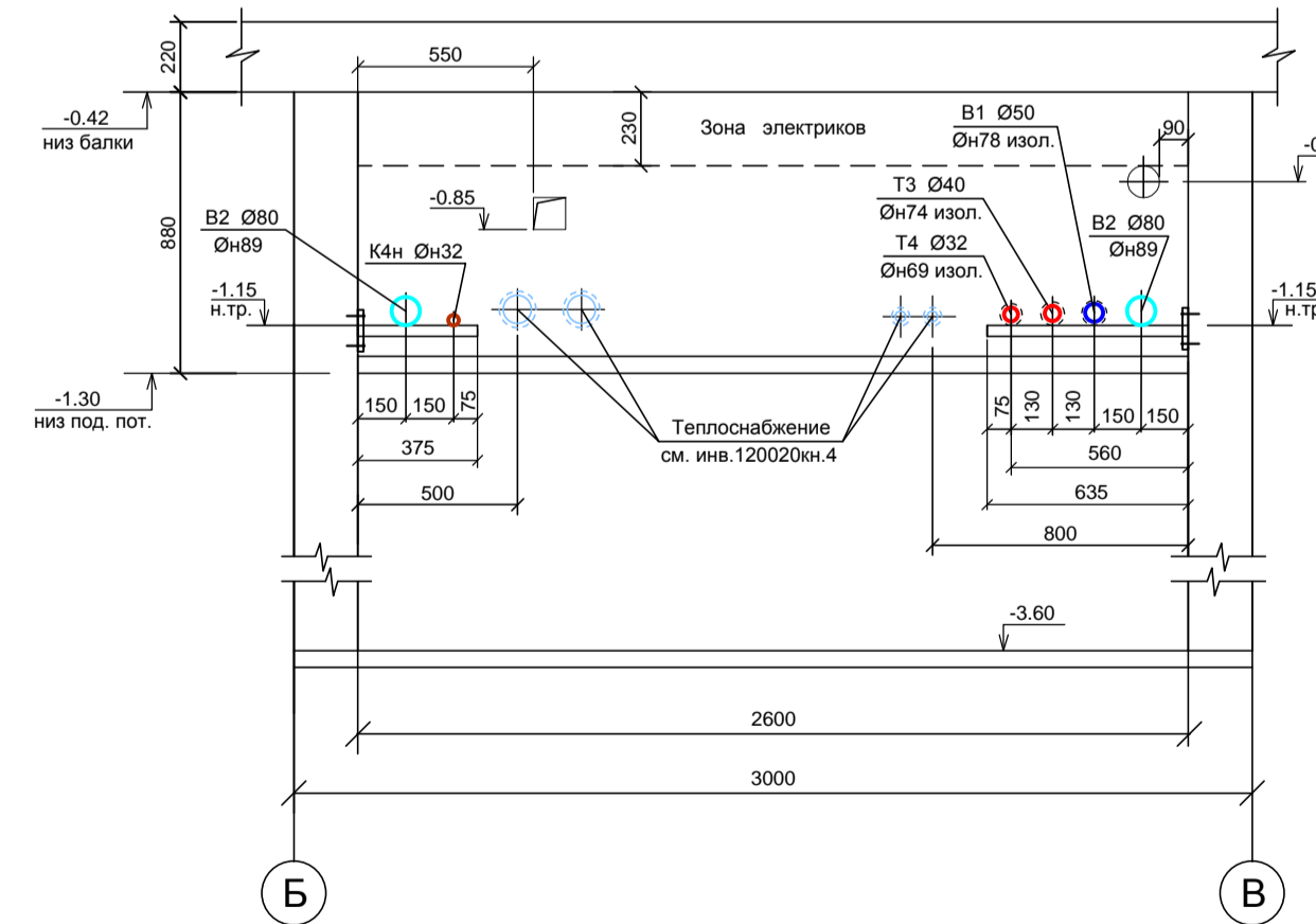
Разрез 2-2 М 1:25
