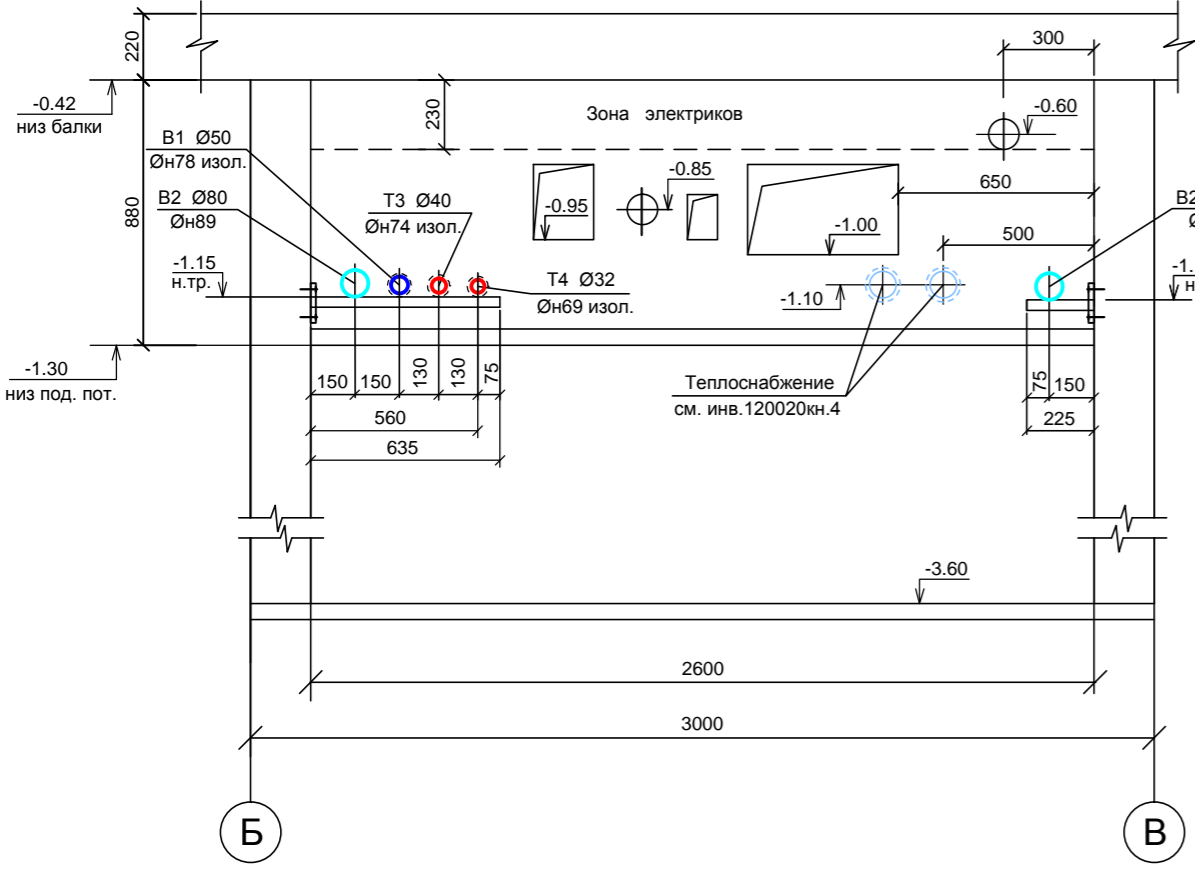
Разрез 3-3 М 1:25
