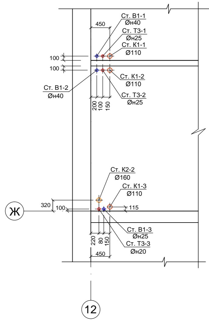
План узла Б М 1:50
