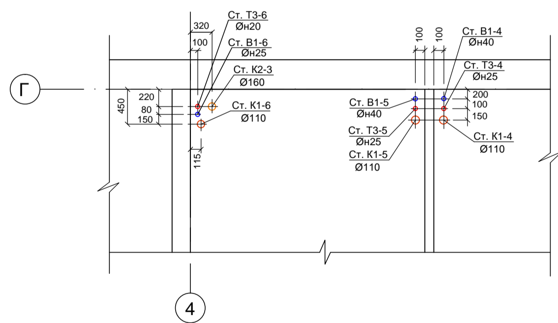
План узла А М 1:50
