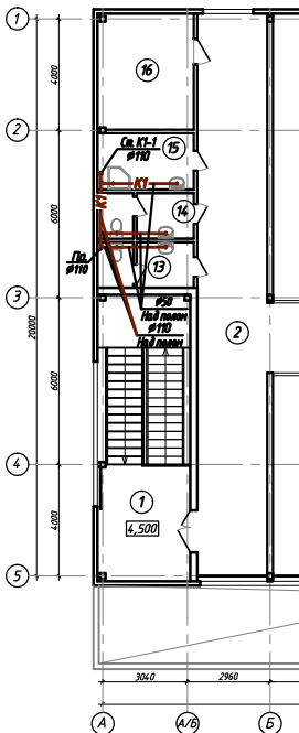
Фрагмент плана 2-го этажа с сетью К1 в осях 1-5 и А-Б. М1:100.
