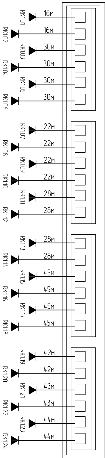
Распределительная панель №1
