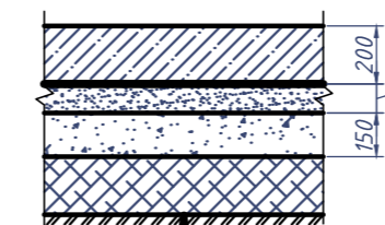
Деталь покрытия площадки компостирования (тип 1)
