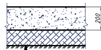
Деталь покрытия грунтовой дороги (тип 2)
