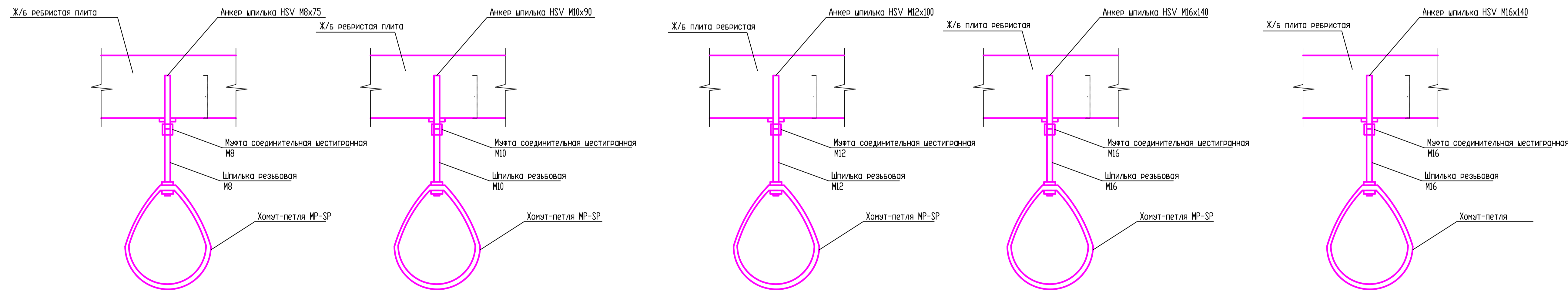
Узел крепления тросопроводов Ø40-50 Узел крепления тросопроводов Ø65-100 Узел крепления тросопроводов Ø150 Узел крепления тросопроводов Ø200 Узел крепления тросопроводов Ø250
