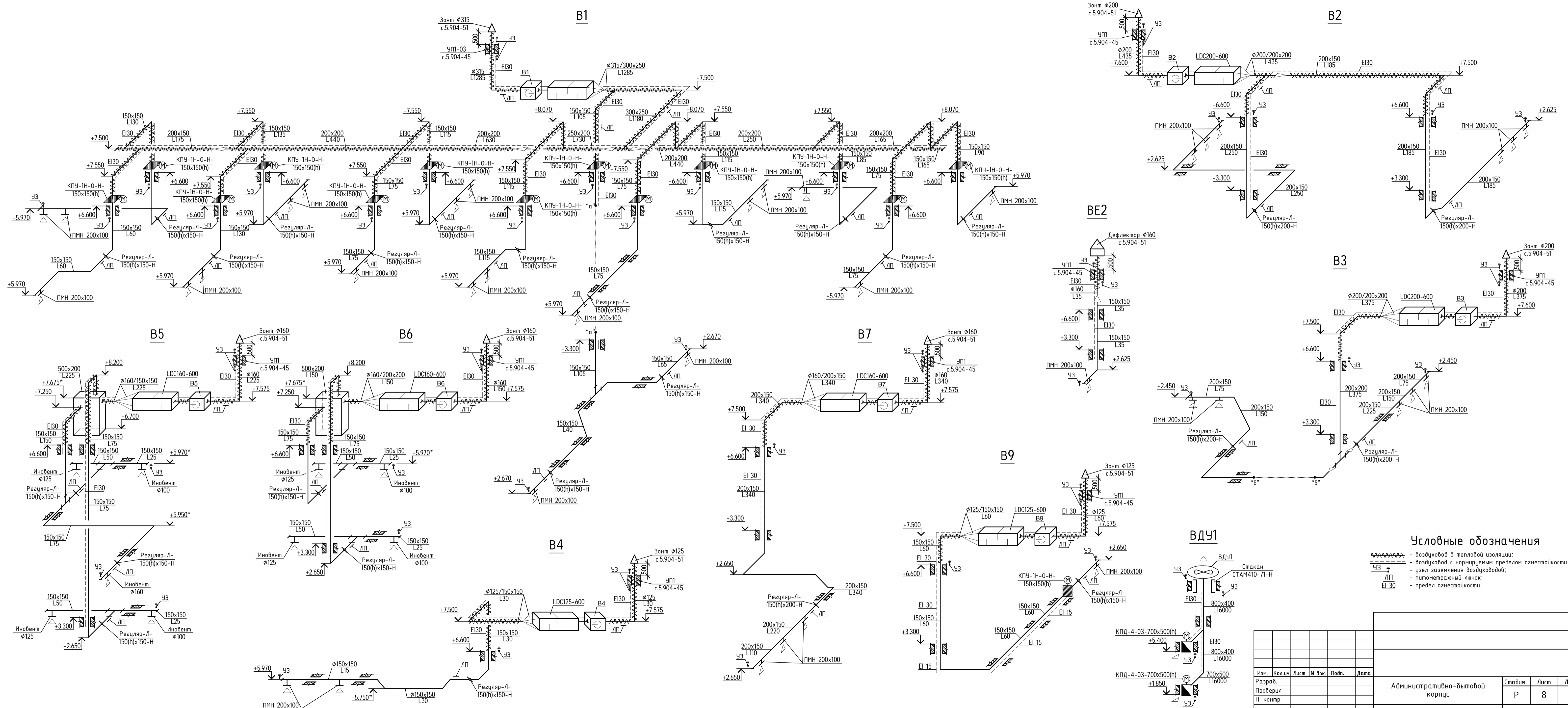
Схемы систем B1-B7, B9, BE2, BДЧ1
