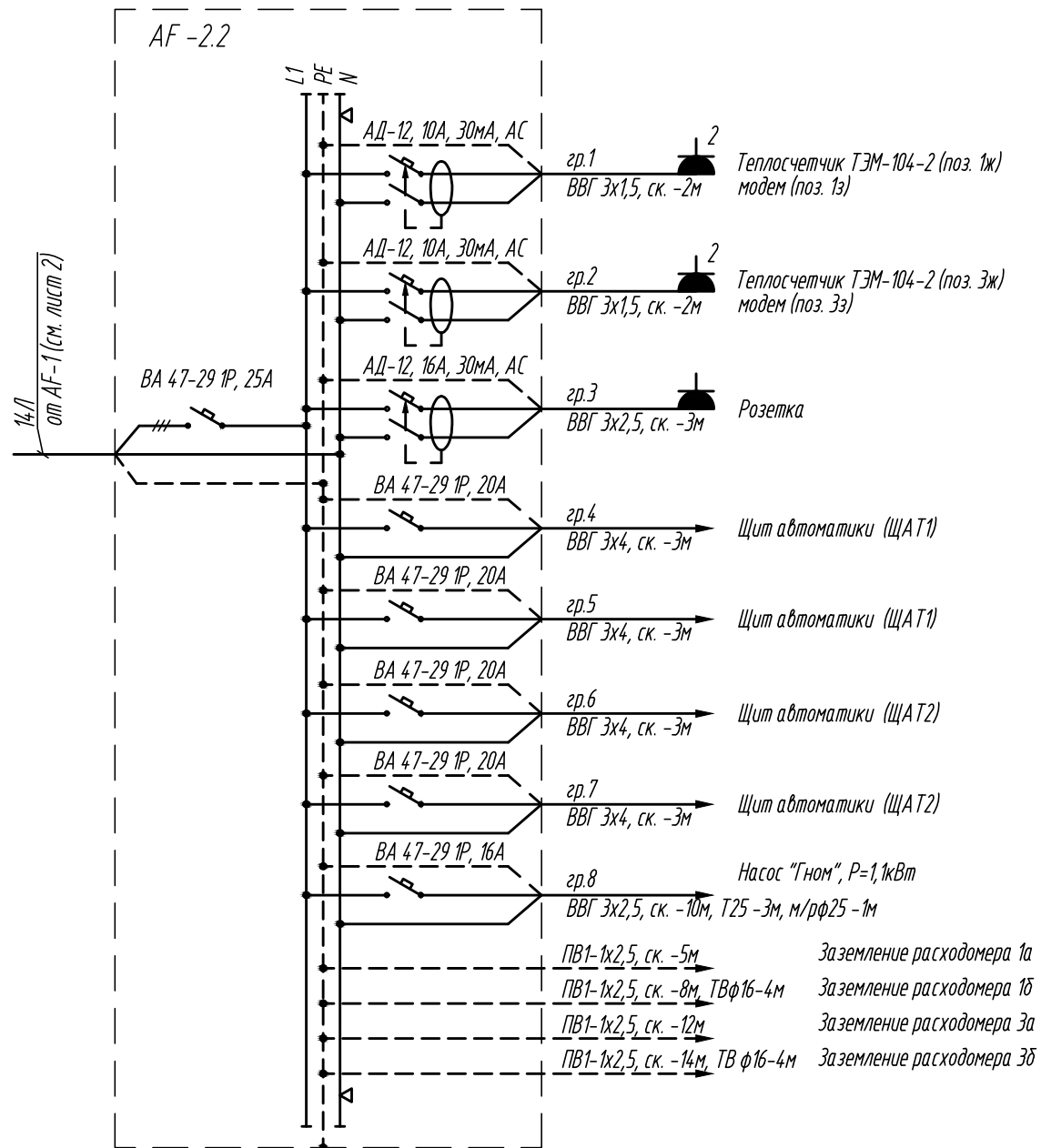
Расчетная схема щита теплового пункта (AF-2.2)
