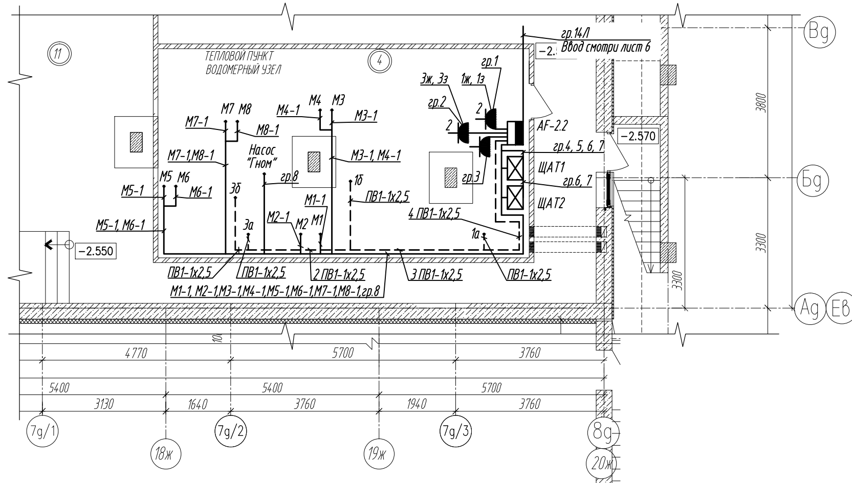
Фрагмент плана подвала в осях Ад-Вд, 7д/1-8д. Тепловой пункт. Силовое электрооборудование.
