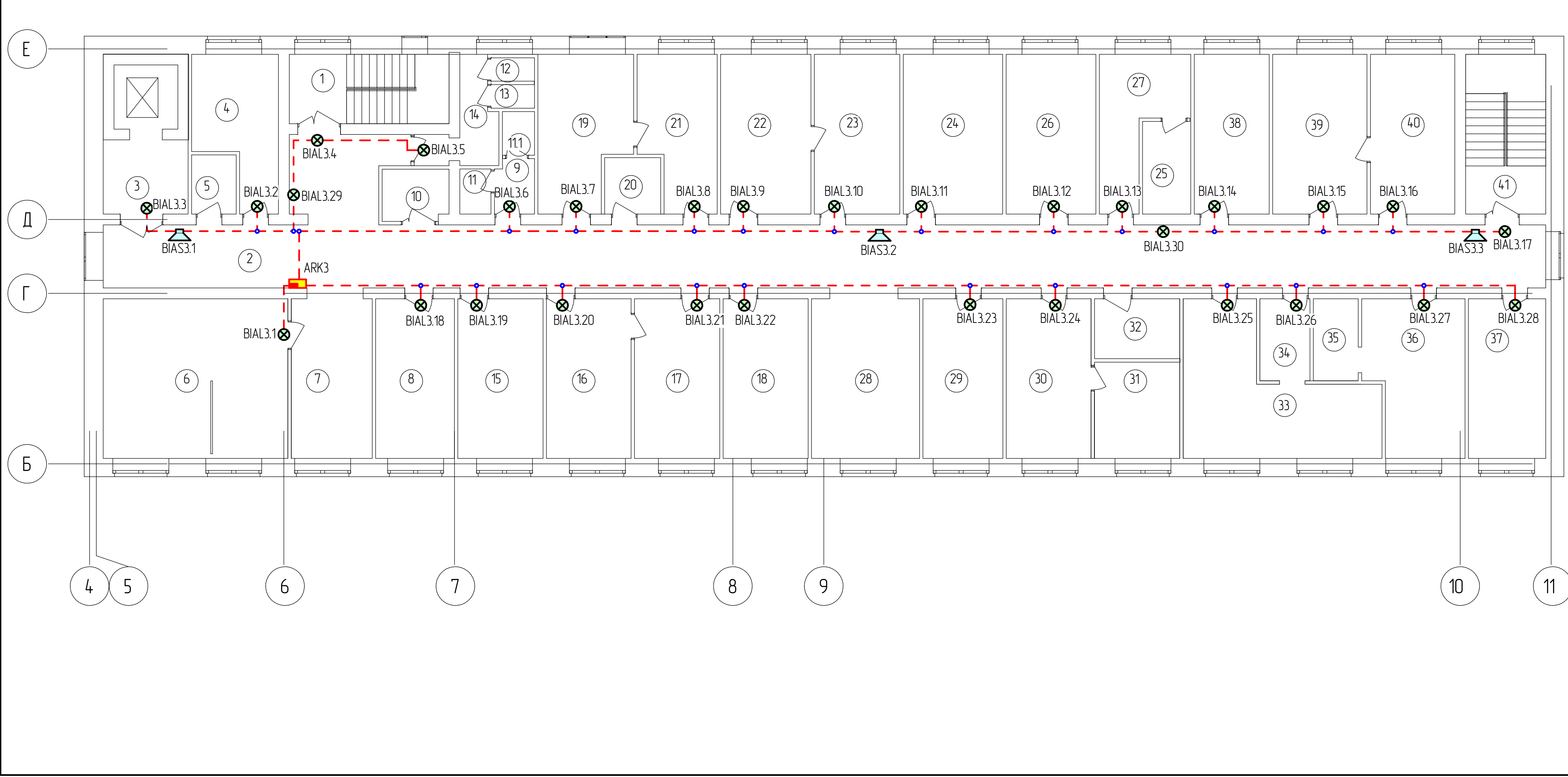
Схема монтажная оповещателей второго этажа. Экспликация помещений
