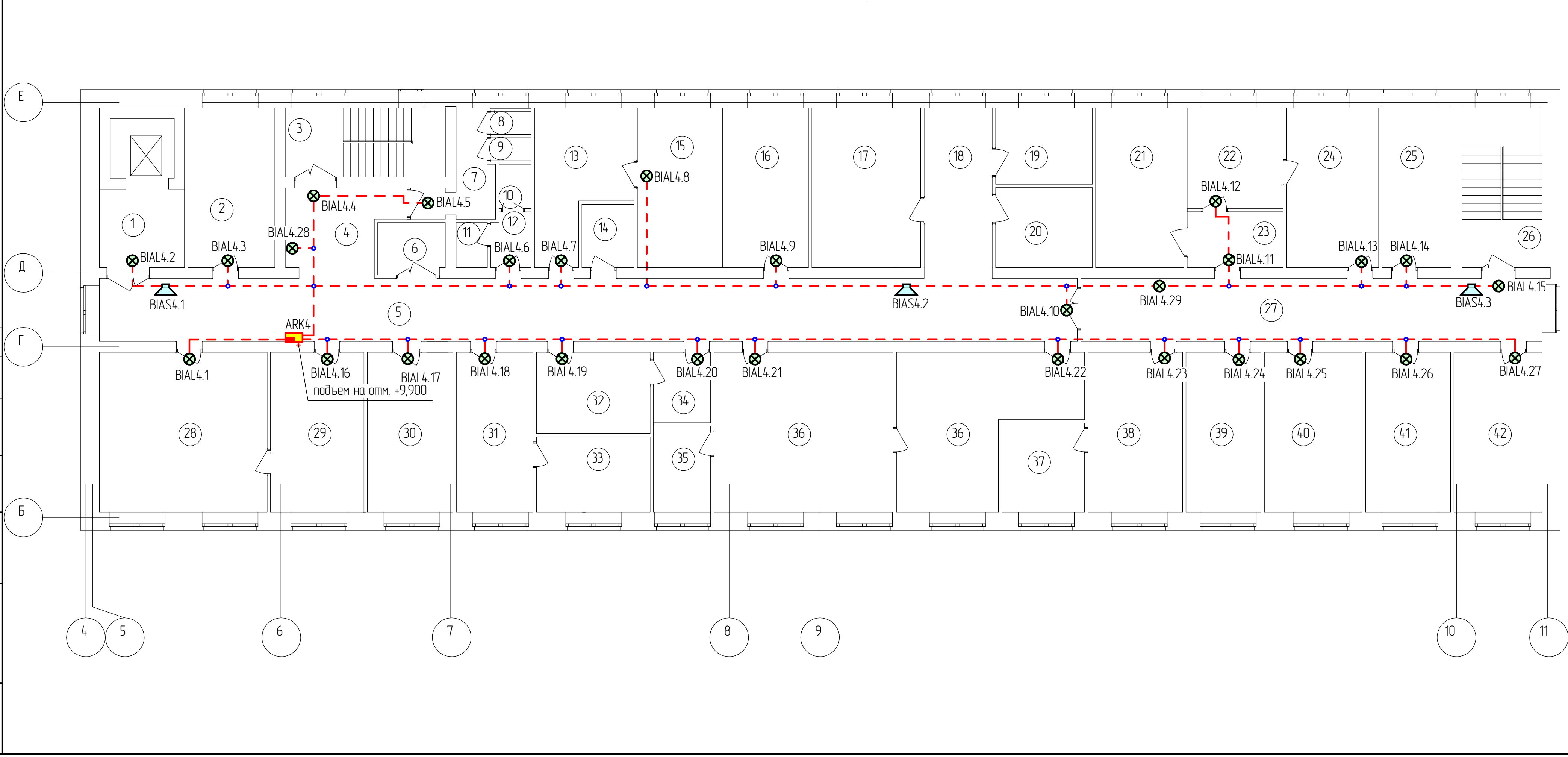
Схема монтажная оповещателей третьего этажа. Экспликация помещений
