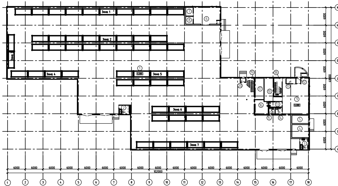
Фрагмент плана 1 этажа
