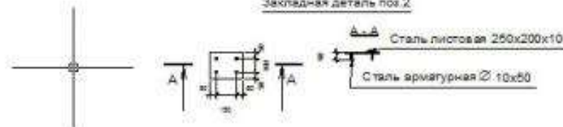
Закладная деталь поз. 2
