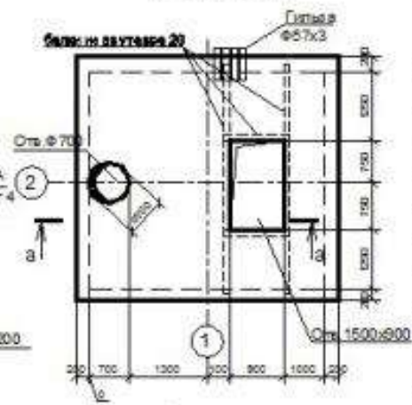
2-2 (к листу 3)
