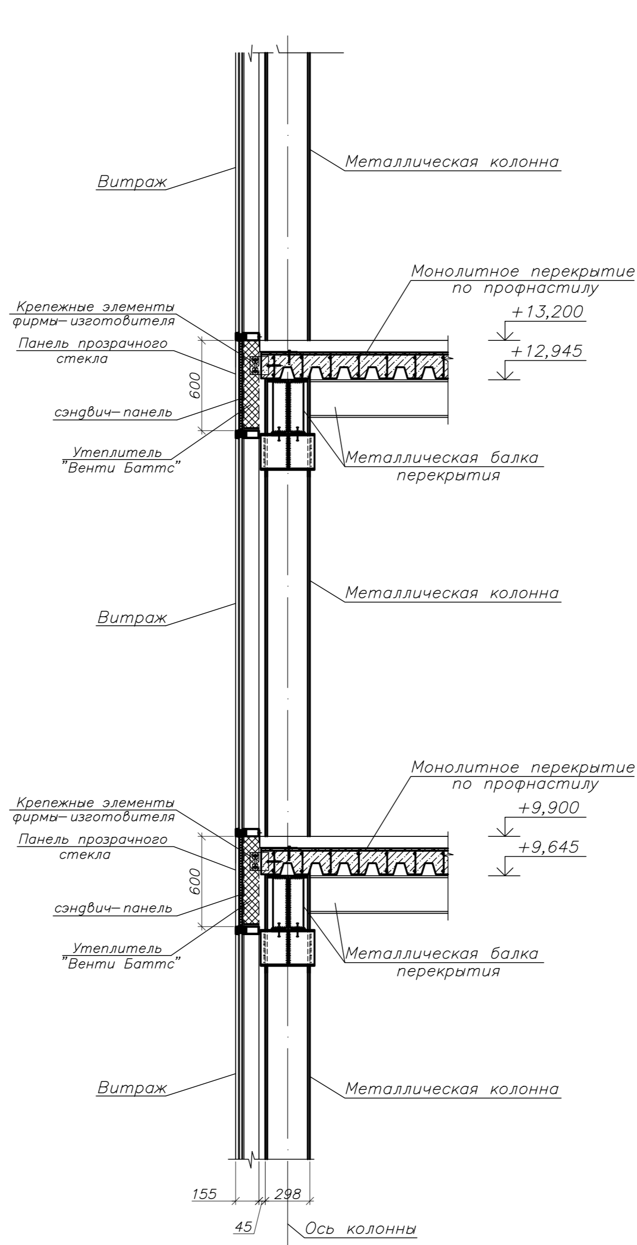
Сечение стены по витражу в круглой части в осях 1-2 (продолжение)
