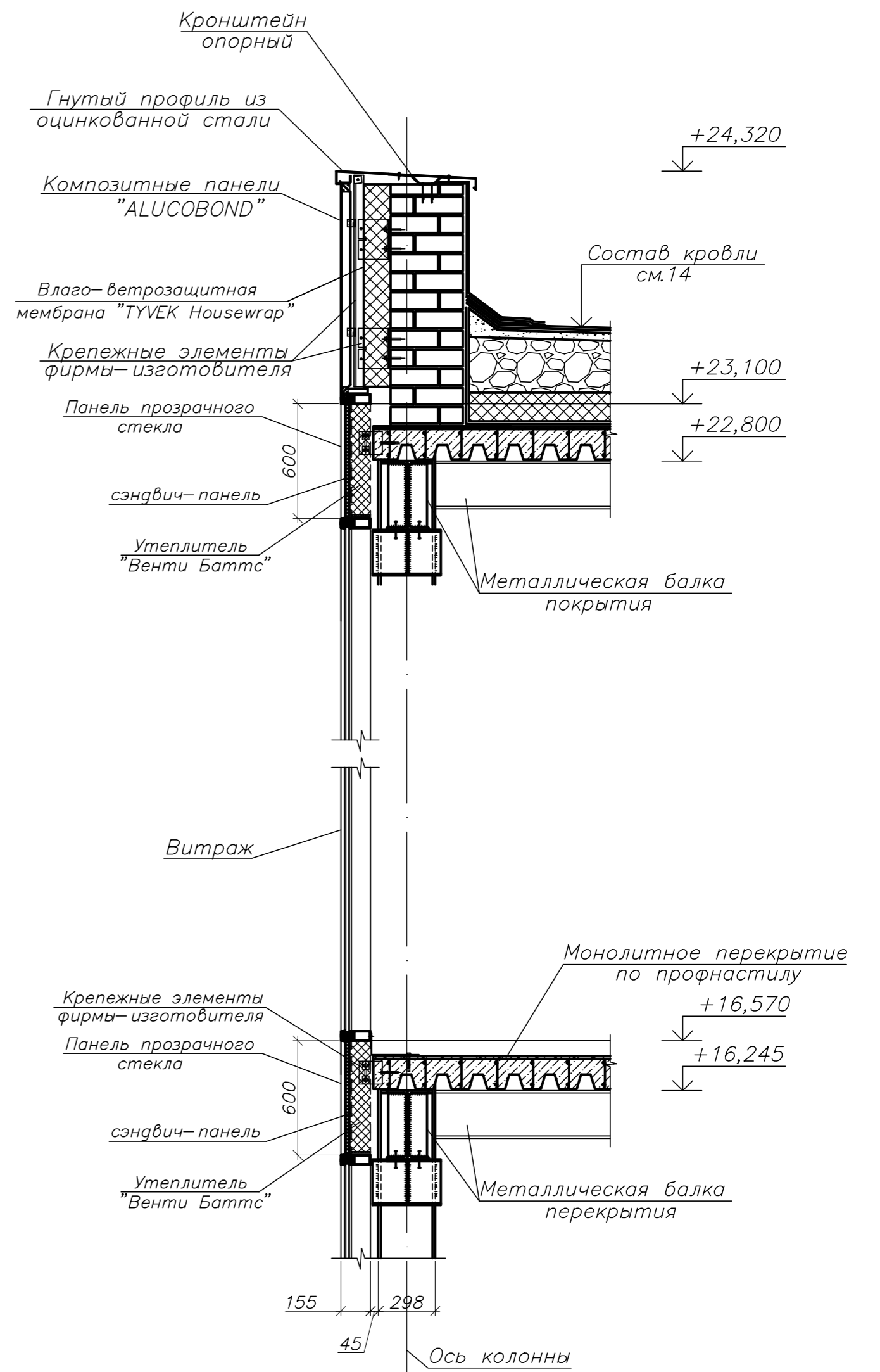
Сечение стены по витражу в круглой части в осях 1-2 (окончание)
