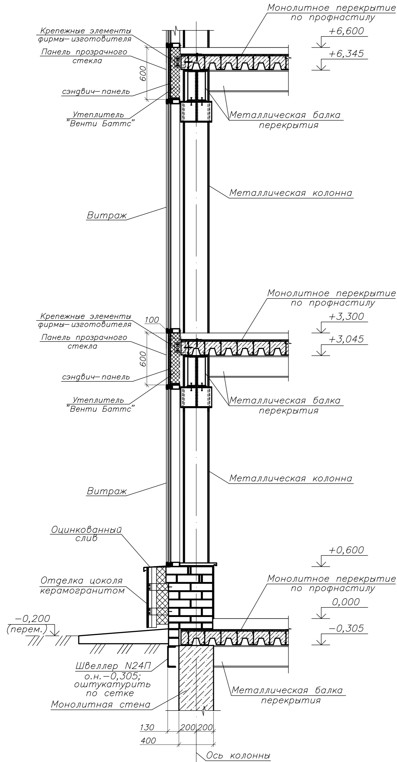
Сечение стены по витражу в круглой части в осях 1-2 (начало)
