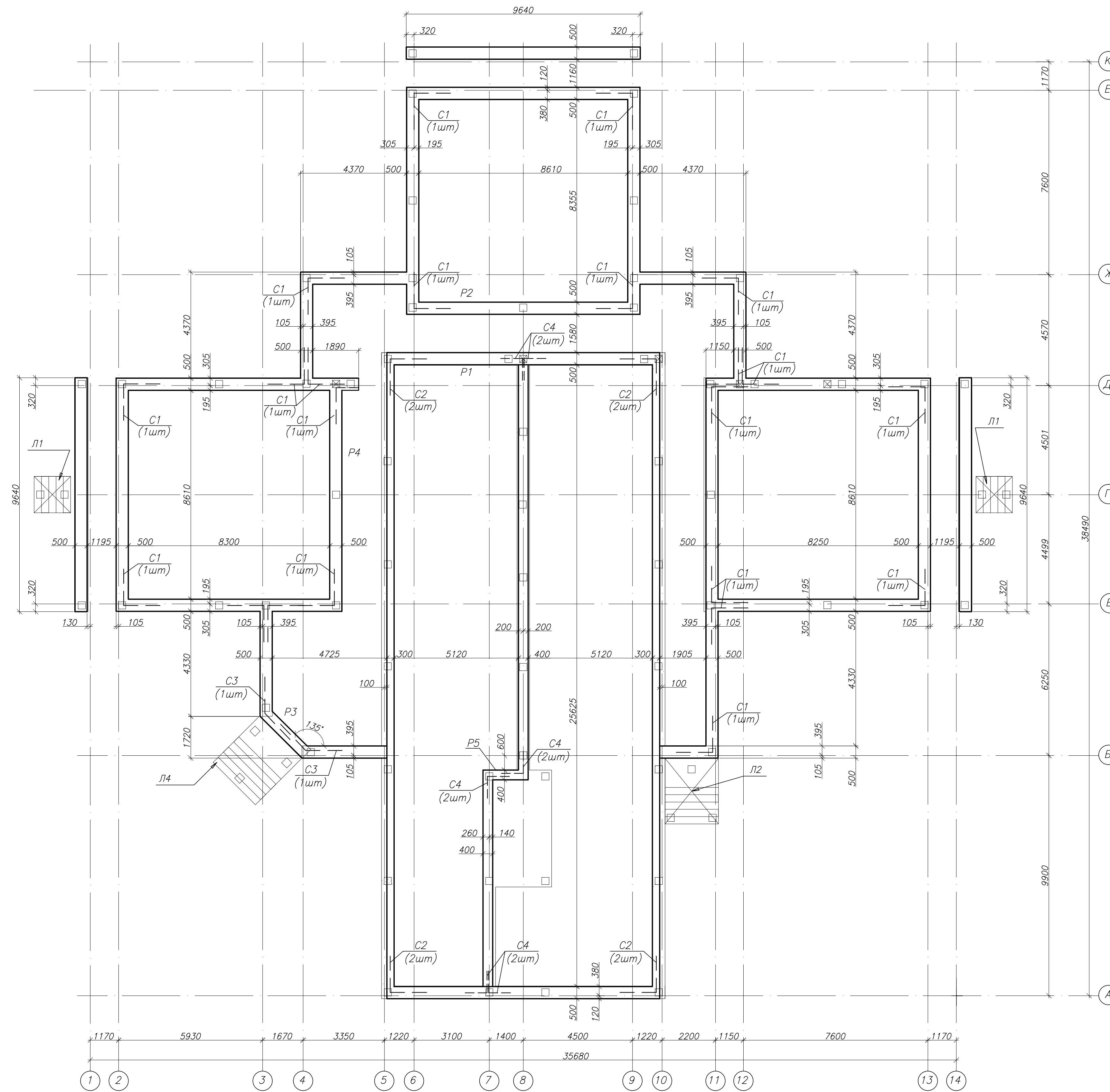
Схема расположения фундаментных блоков
