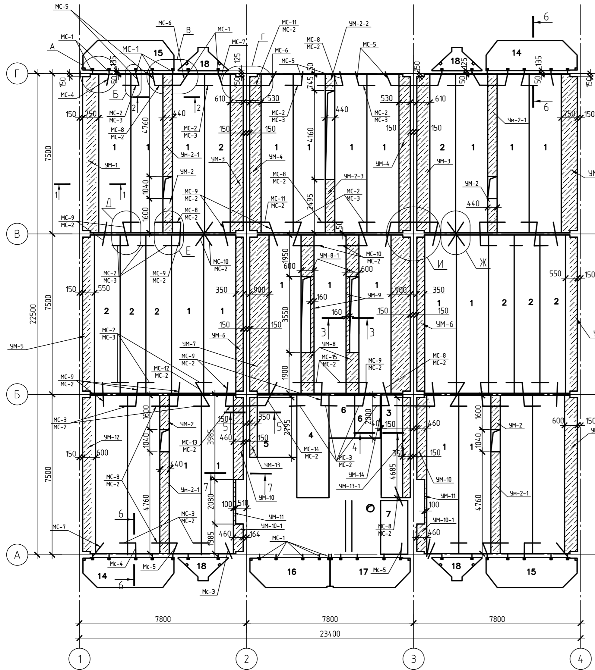
Монтажная схема перекрытия цокольного этажа
