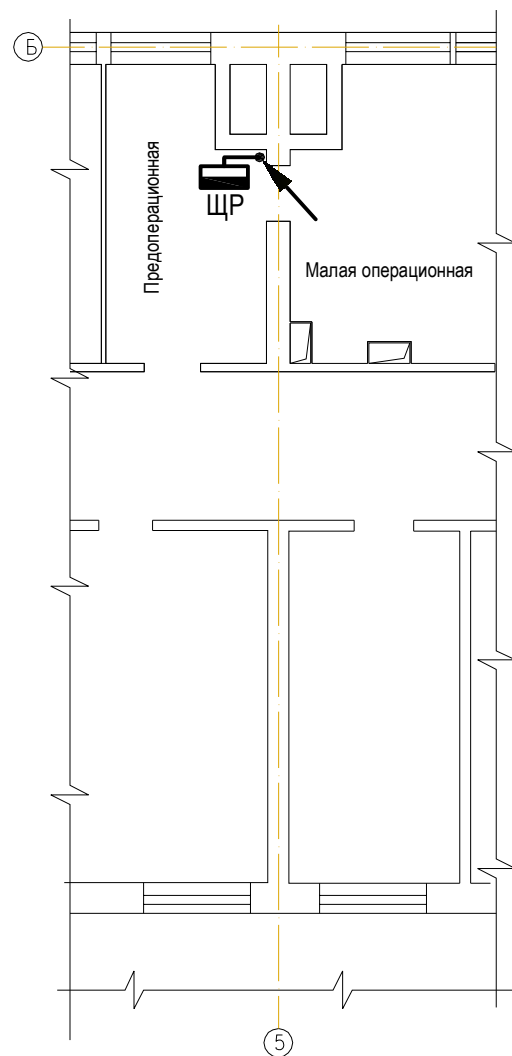
План 1 этажа. М 1:125.
