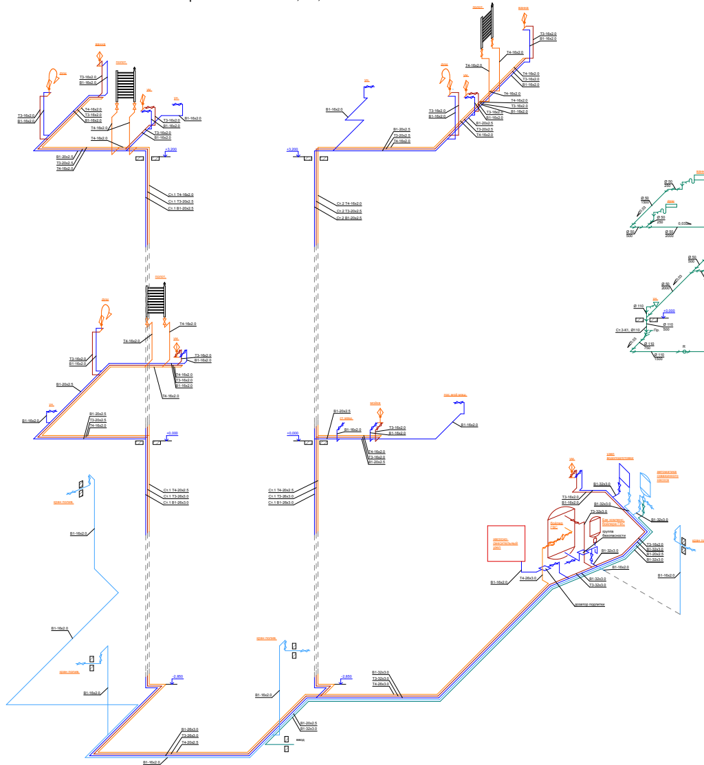
АксонOMETрическая схема В1, Т3, Т4.
