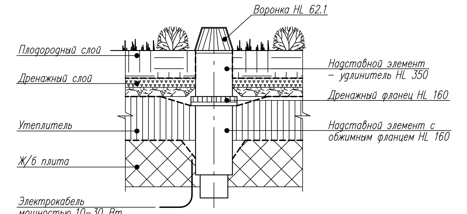
Рисунок 1 Установка воронки Н. 62.1 с электрообогревом на эксплуатируемой кровле
