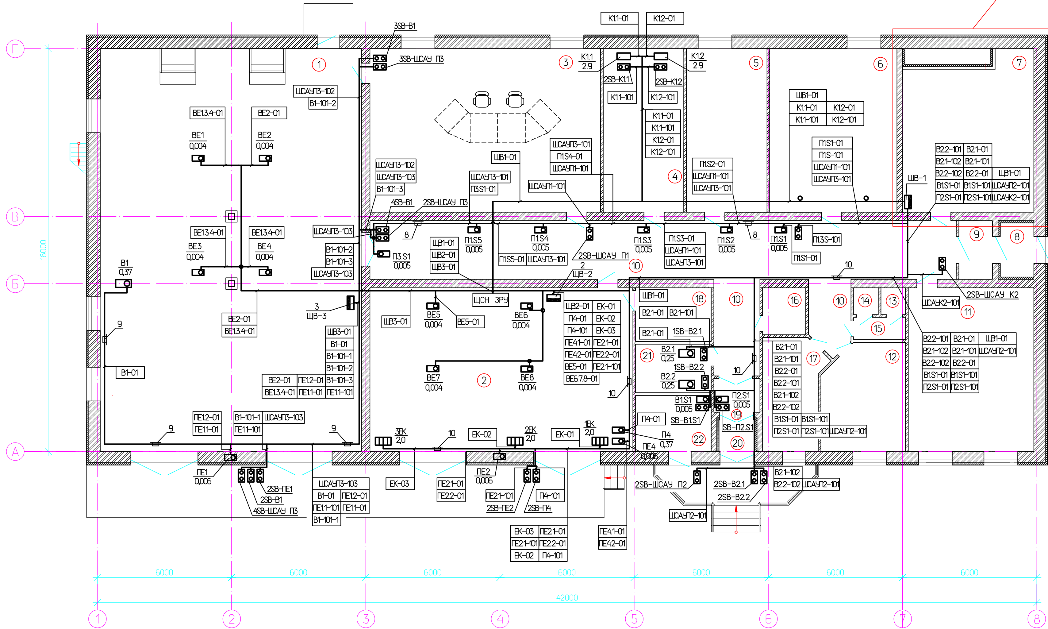
План на отм. 0.000 Масштаб 1:100
