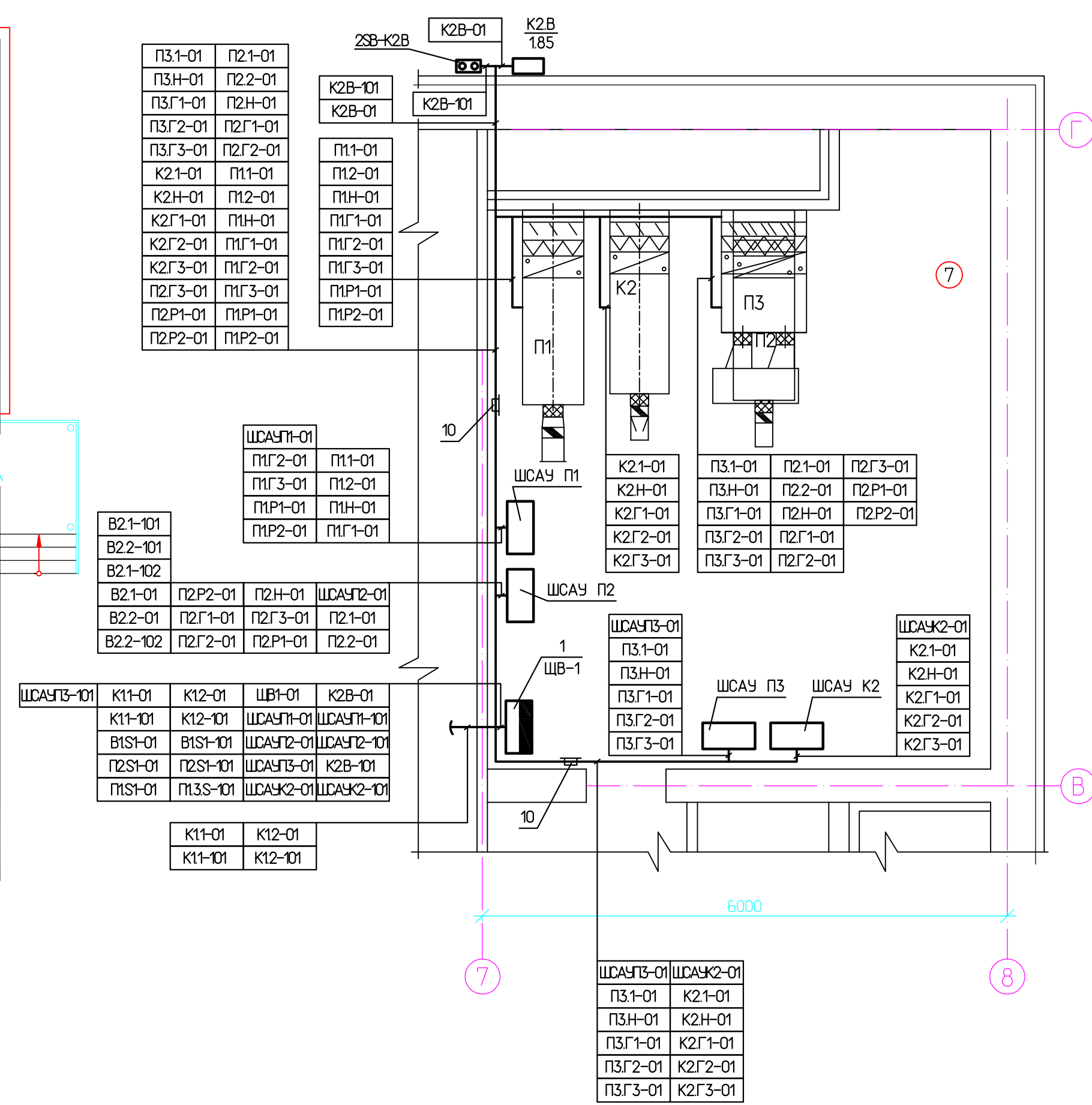
План на отм. 0.000 Масштаб 1:50
