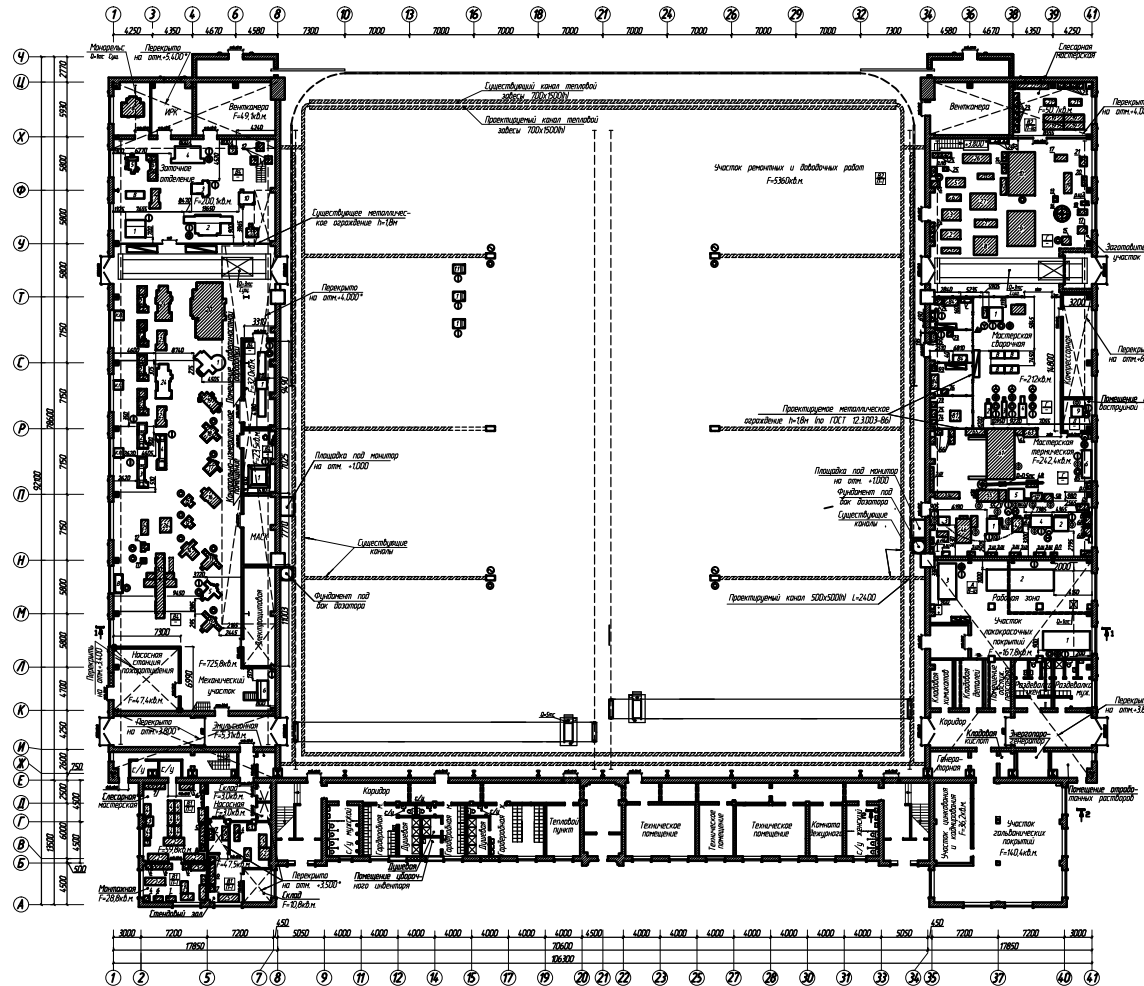
План 1-го этажа М 1:200
