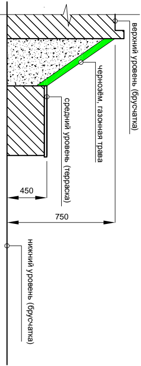
Сечение 2-2
