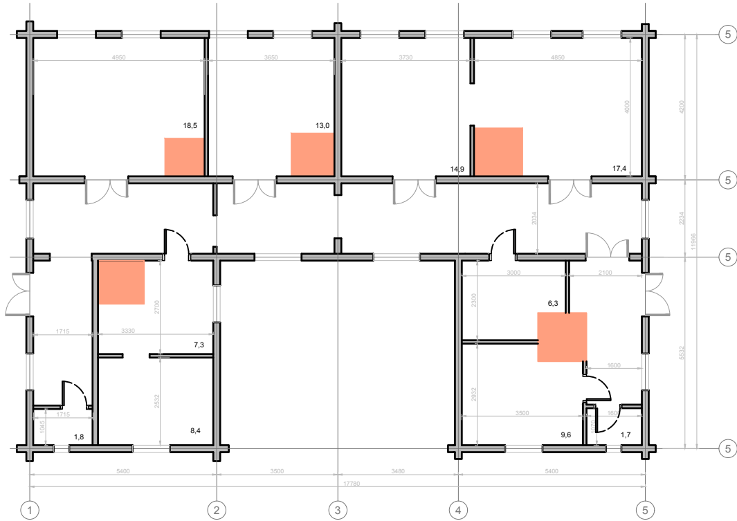
План на отм. 0.000 (существующий) М 1:150
