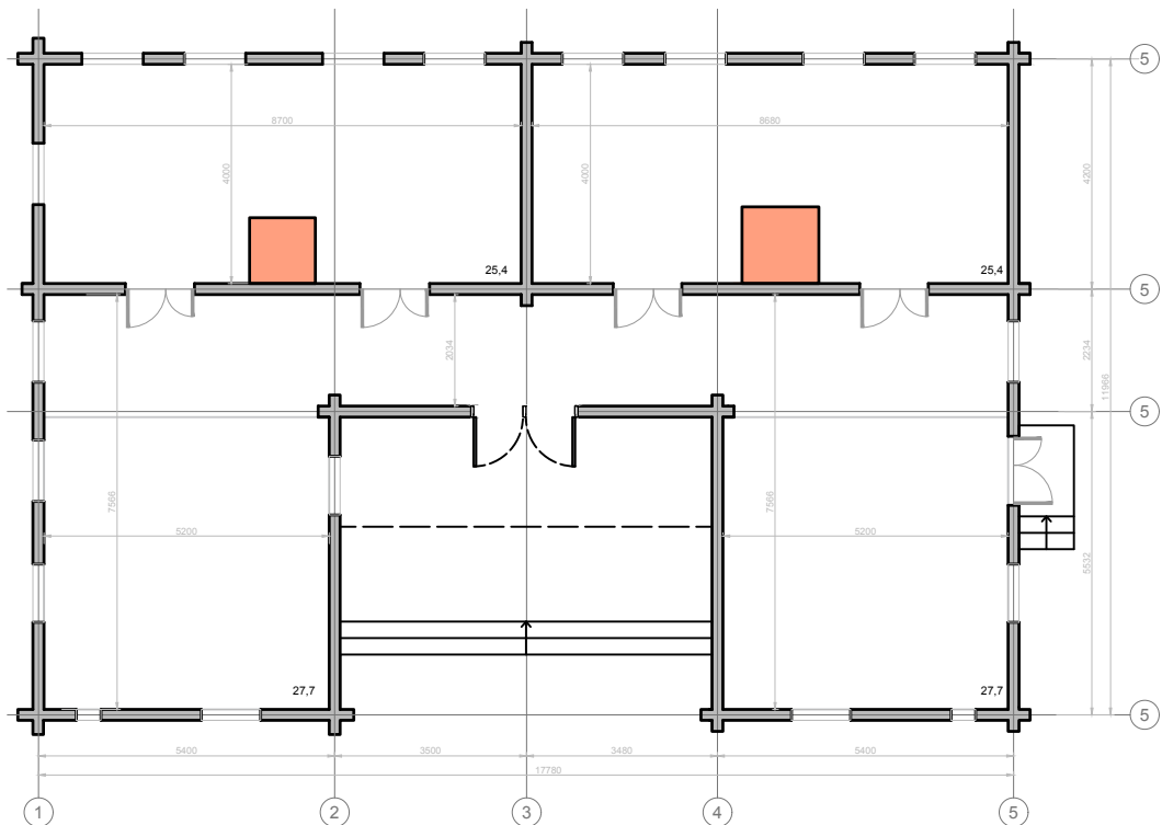
План на отм. 0.000 (проектный) М 1:150
