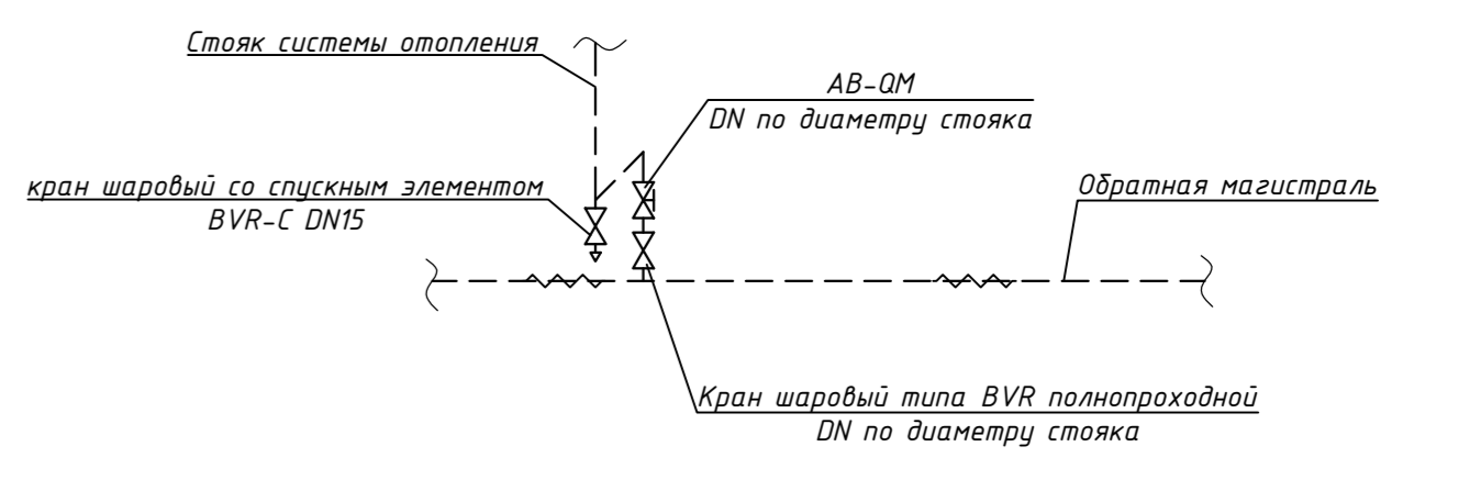
Узел присоединение стоек к обратной магистрали T2
