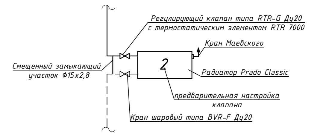
Узел обвязки радиатора
