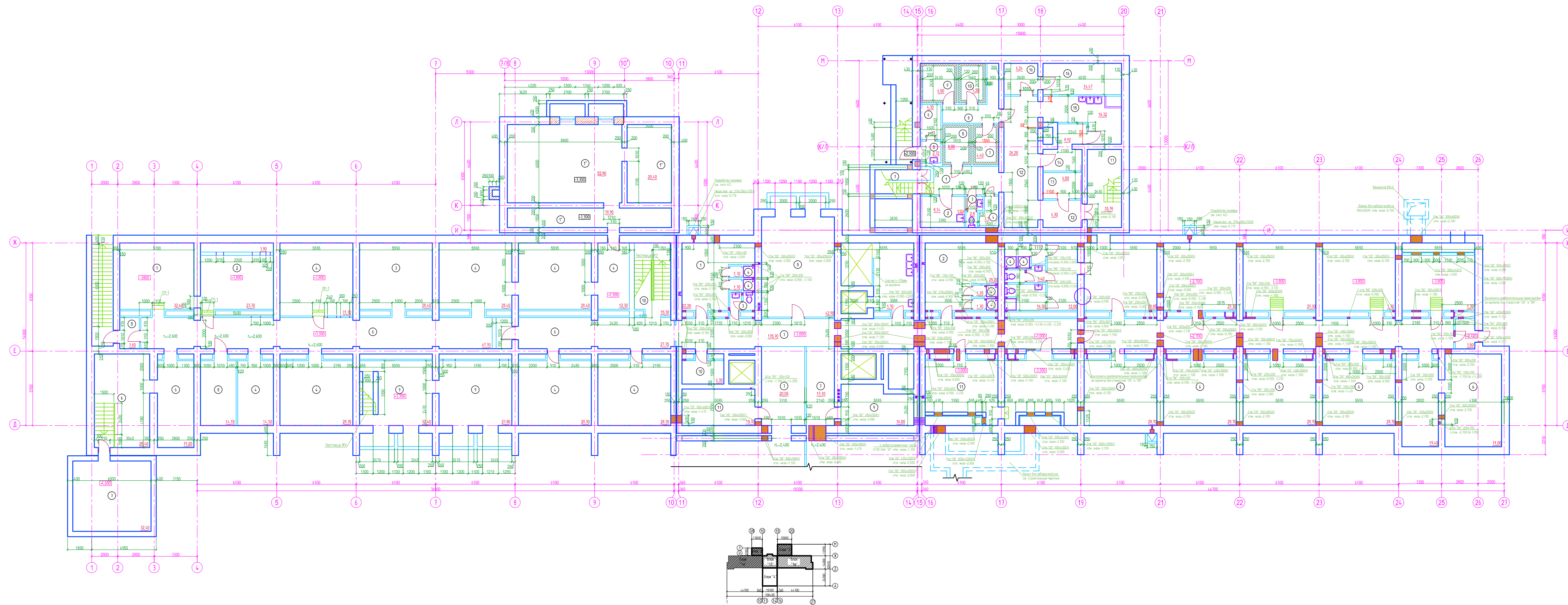
ПЛАН ПОДВАЛА НА ОТМ. -3,000 В ОСЯХ "1-27" ПОСЛЕ РЕКОНСТРУКЦИИ
