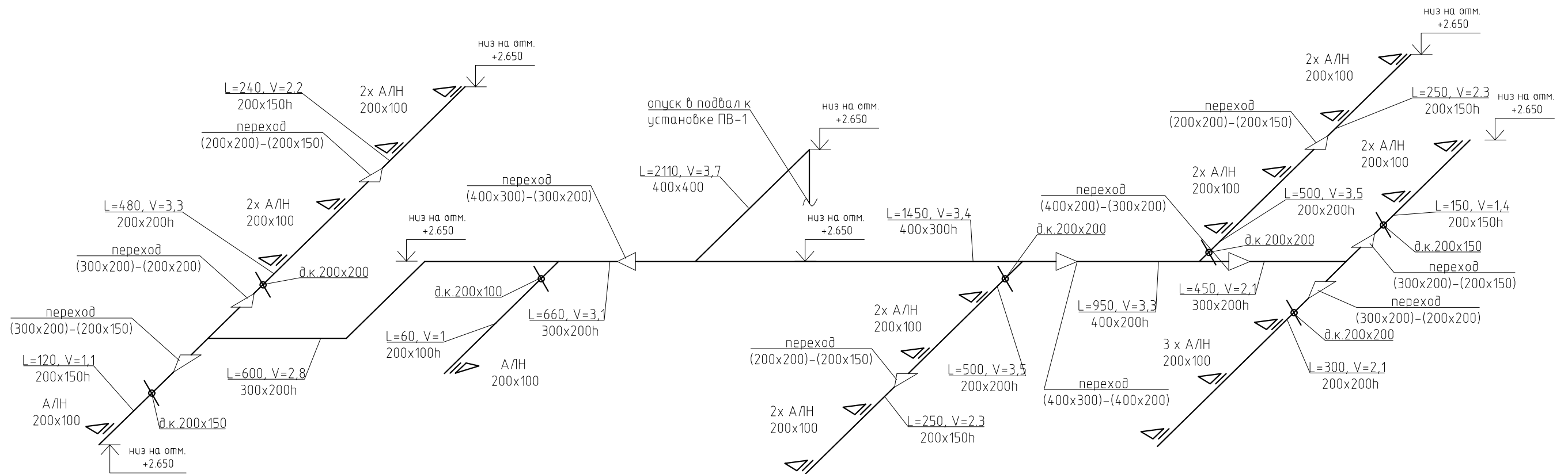
Схема системы ПВ1-П (на 1-м этаже).
