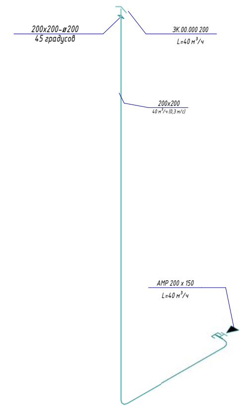
Схема системы ВЕ-2
