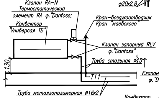
2 Узел обвязки отопительного прибора в совмещенных санузлах
