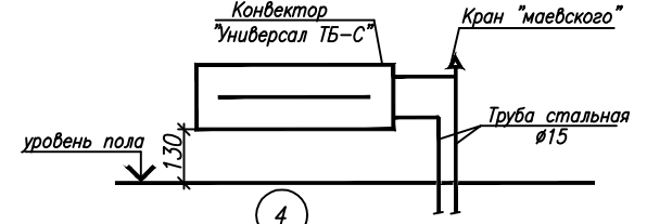
4 Узел обвязки отопительного прибора в ванных комнатах и санузлах
