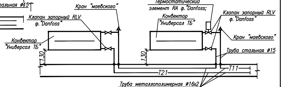
4 Узел обвязки отопительного прибора в ванных комнатах и санузлах
