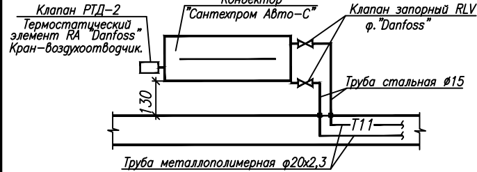
1 Узел обвязки отопительного прибора в квартирах
