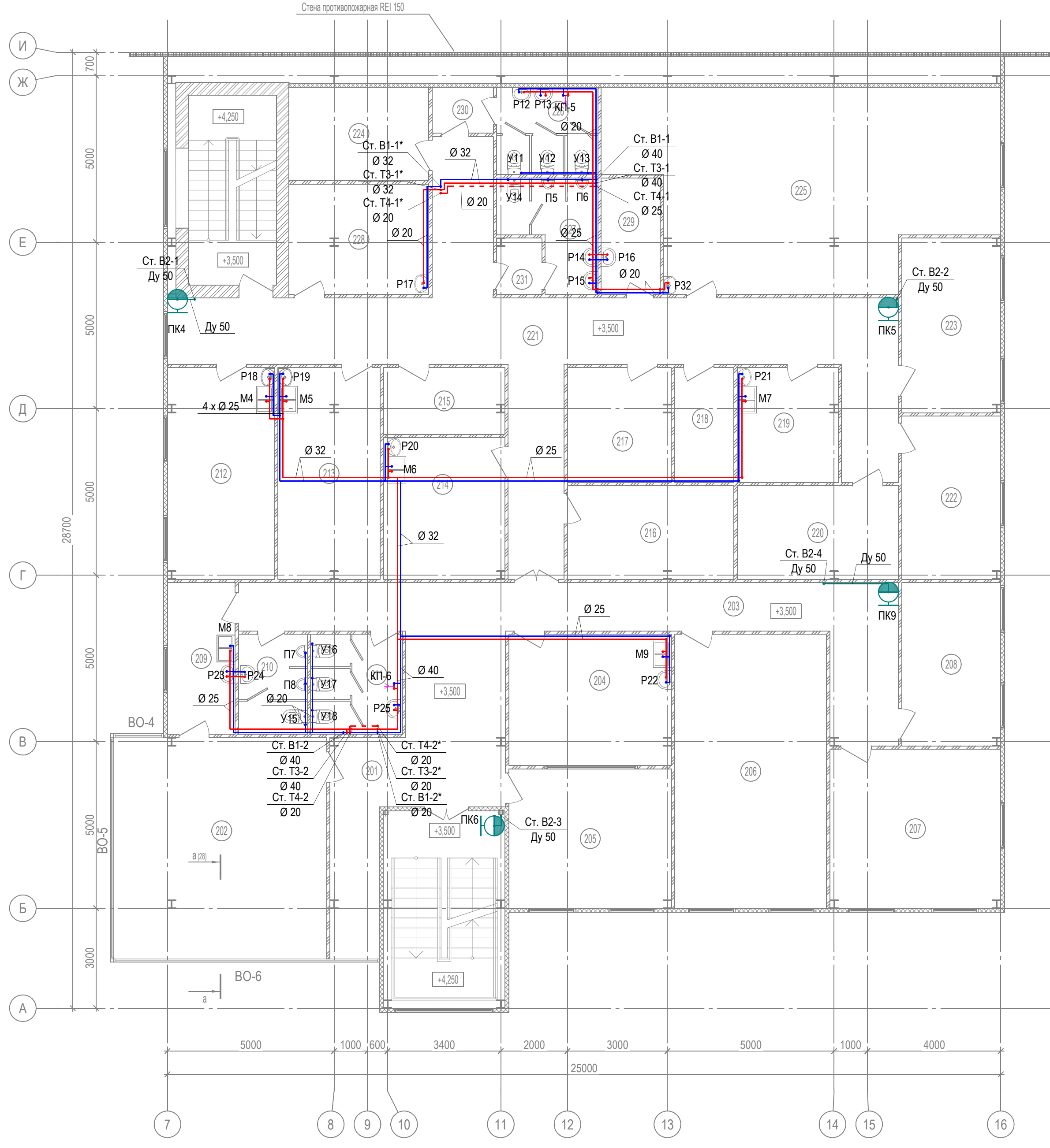
План на отм. +3.500
