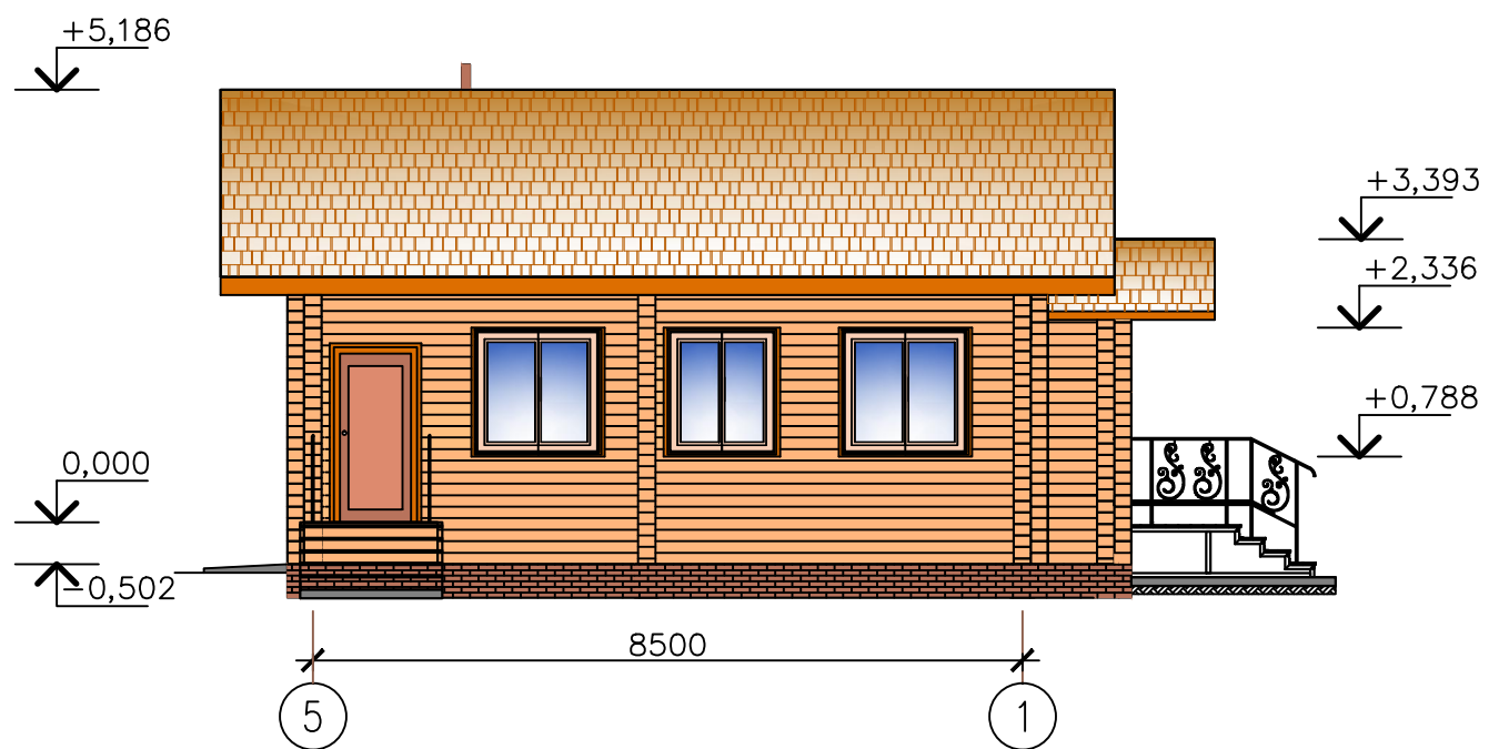
Фасад 5-1
