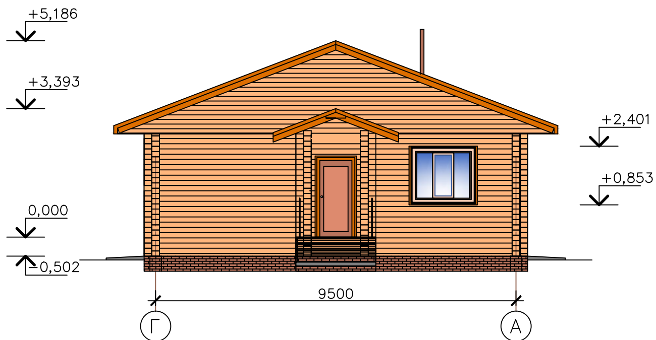
Фасад Г-А
