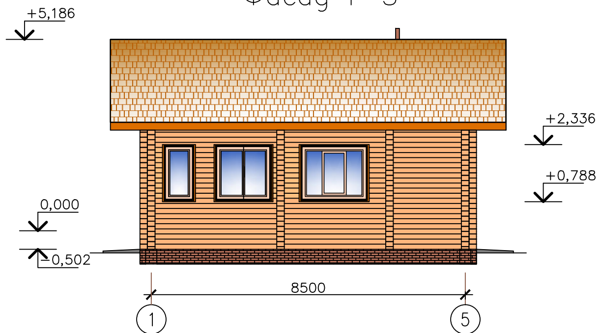
Фасад 1-5
