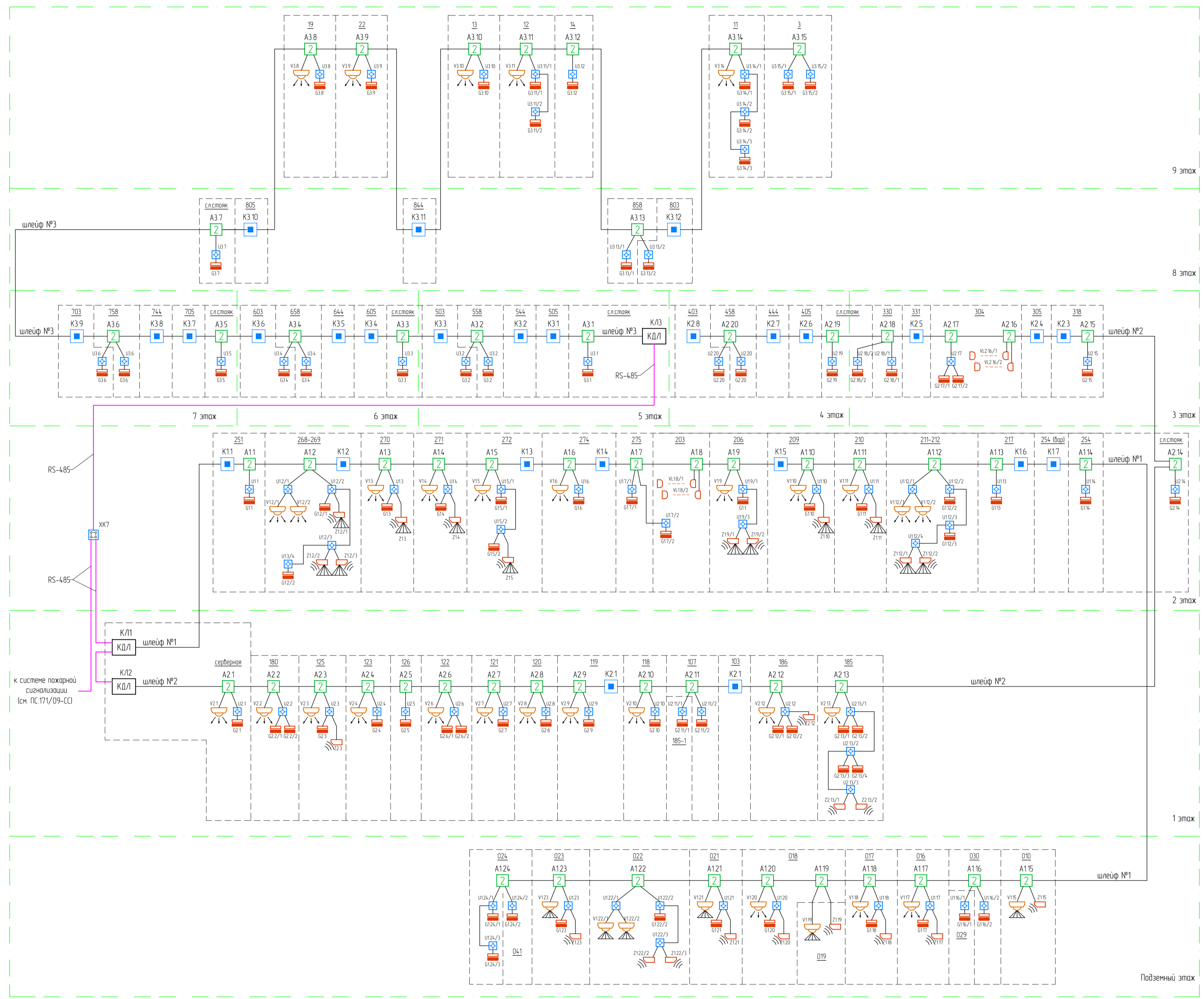
Структурная схема охранных шлейфов
