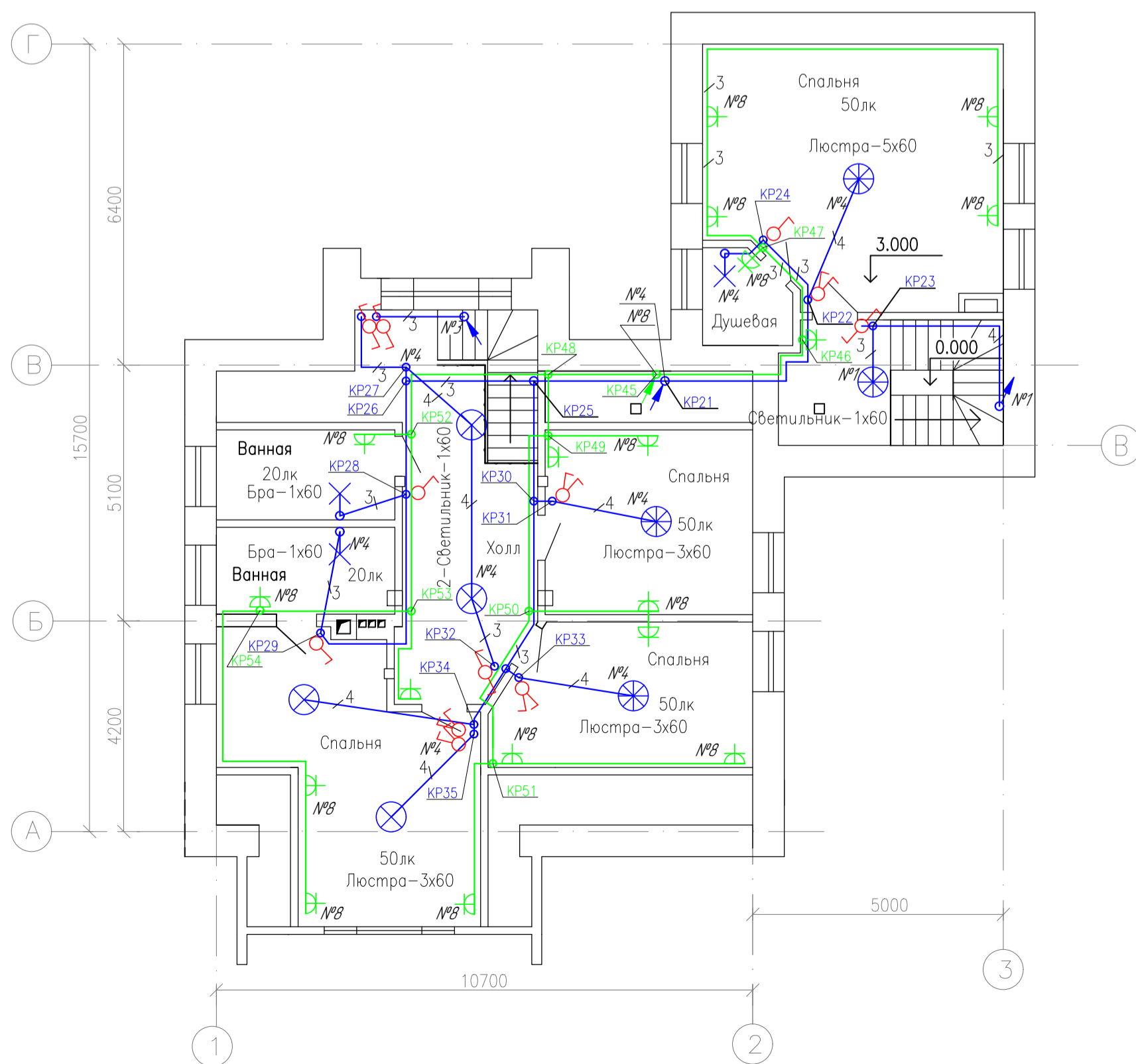
ПЛАН НА ОТМ. 3.000
