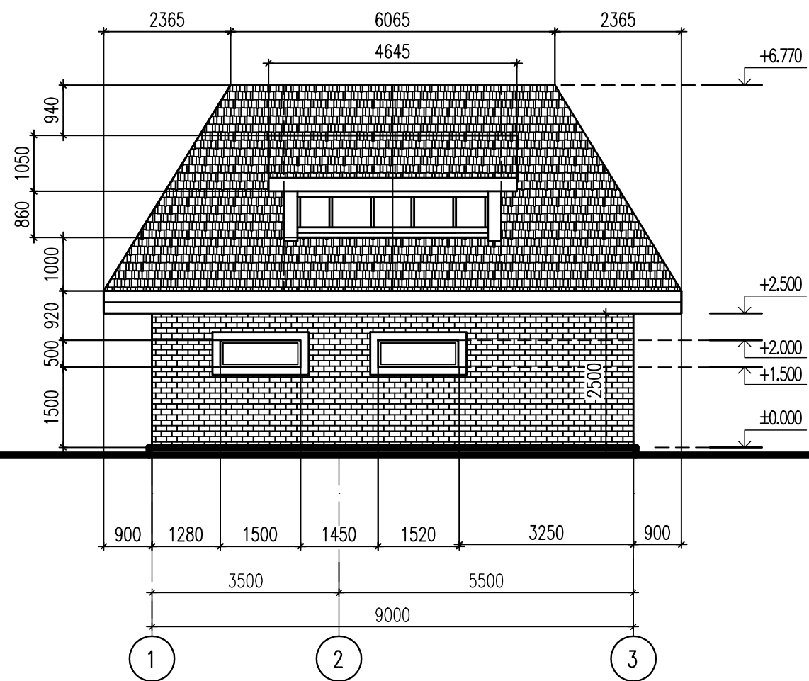
Фасад в осях 1-3
