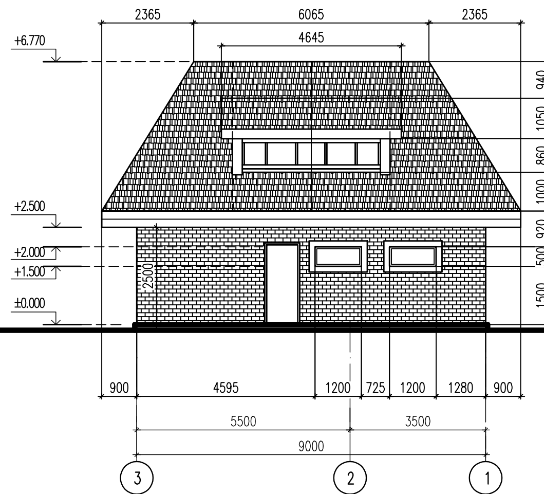
Фасад в осях 3-1
