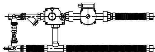
Смесительный узел
