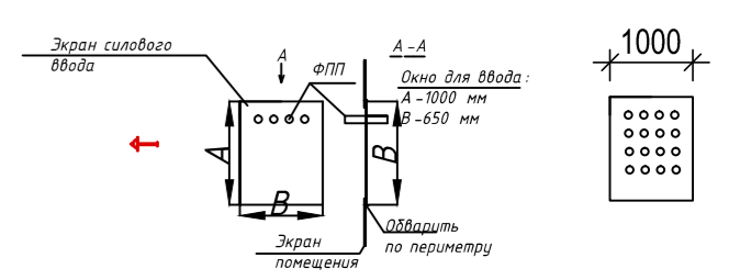
Эскиз типовой установки Силового ввода с ФПП
