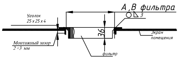
Эскиз типовой установки воздушного фильтра
