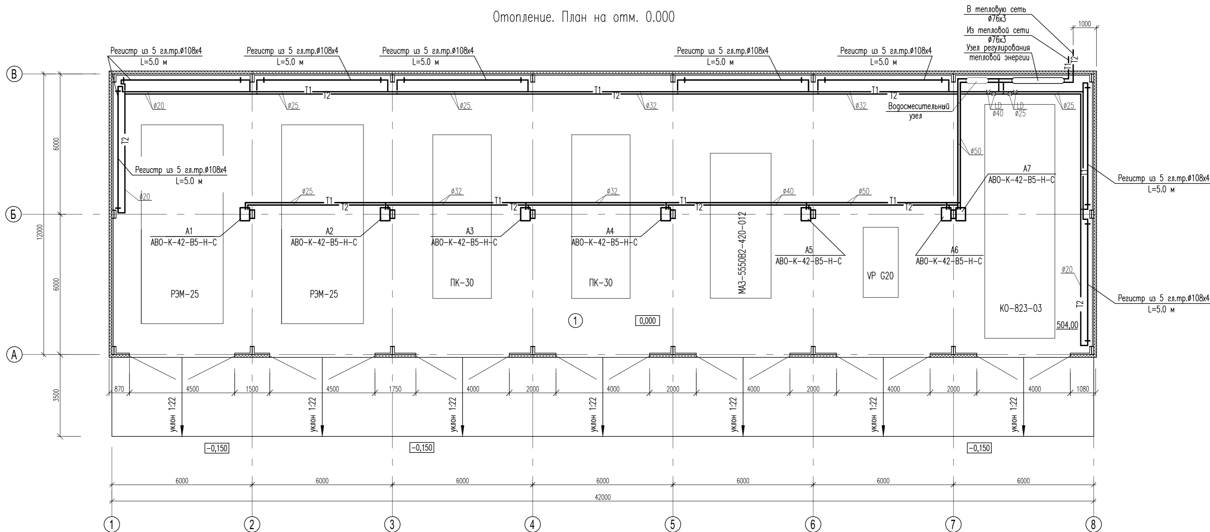
Теплопотери в помещении гаража
