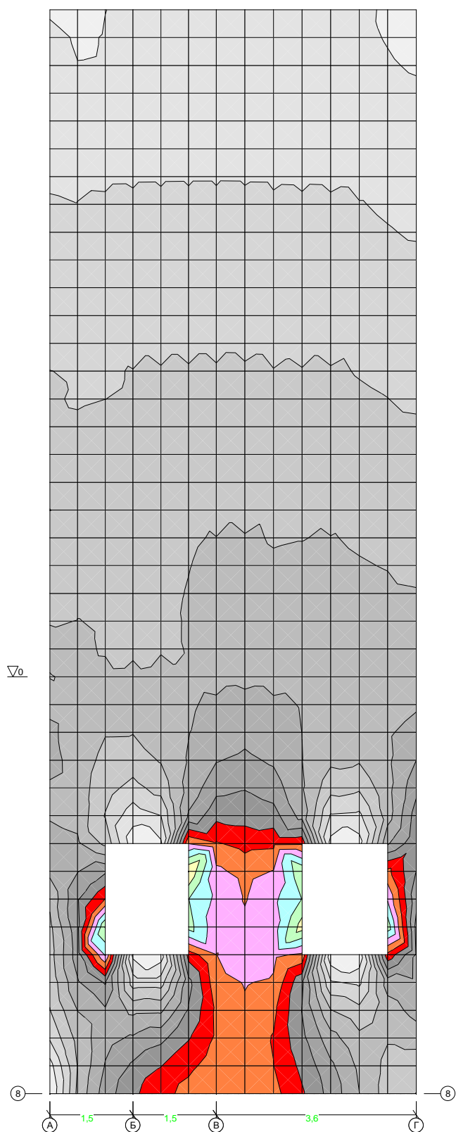
Корпус 13. Стена по оси "8". Вертикальные усилия N.
