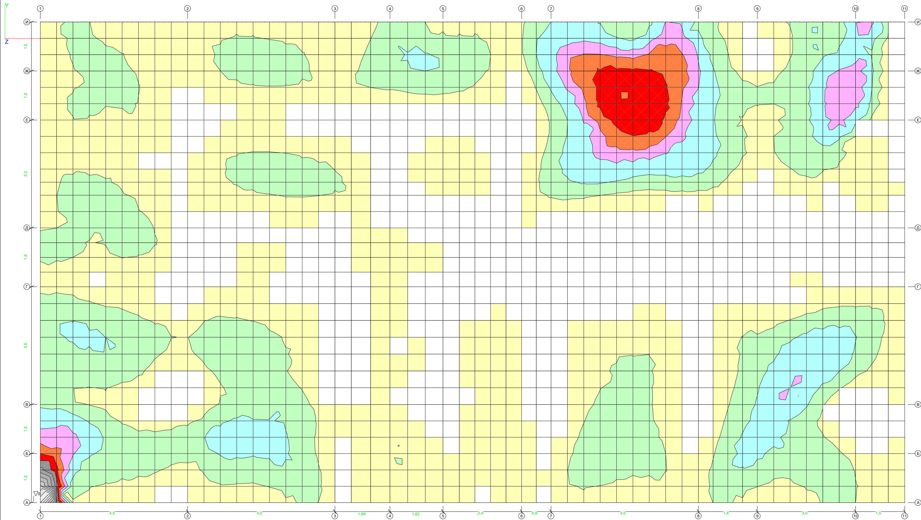
Корпус 13. Фундаментная плита. Армирование. Верхняя по Y
