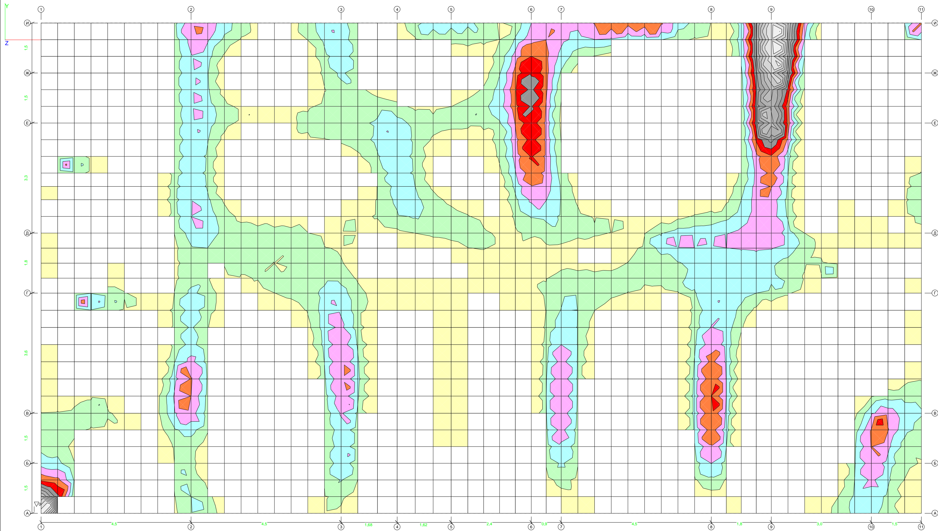
Корпус 13. Фундаментная плита. Армирование. Нижняя по X
